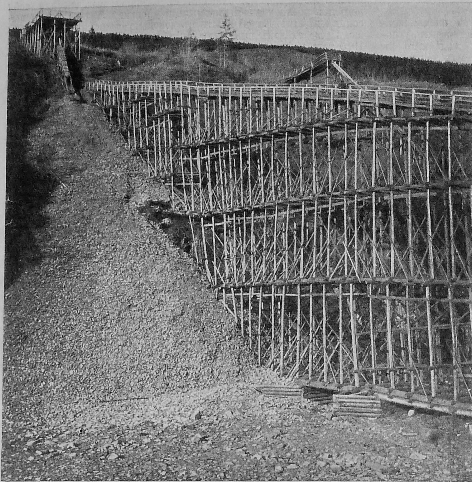
Пріискъ Сисина по рѣчкѣ Хомолхо. Сооруженіе для спуска золотиносныхъ песковъ съ горы для промывки.
