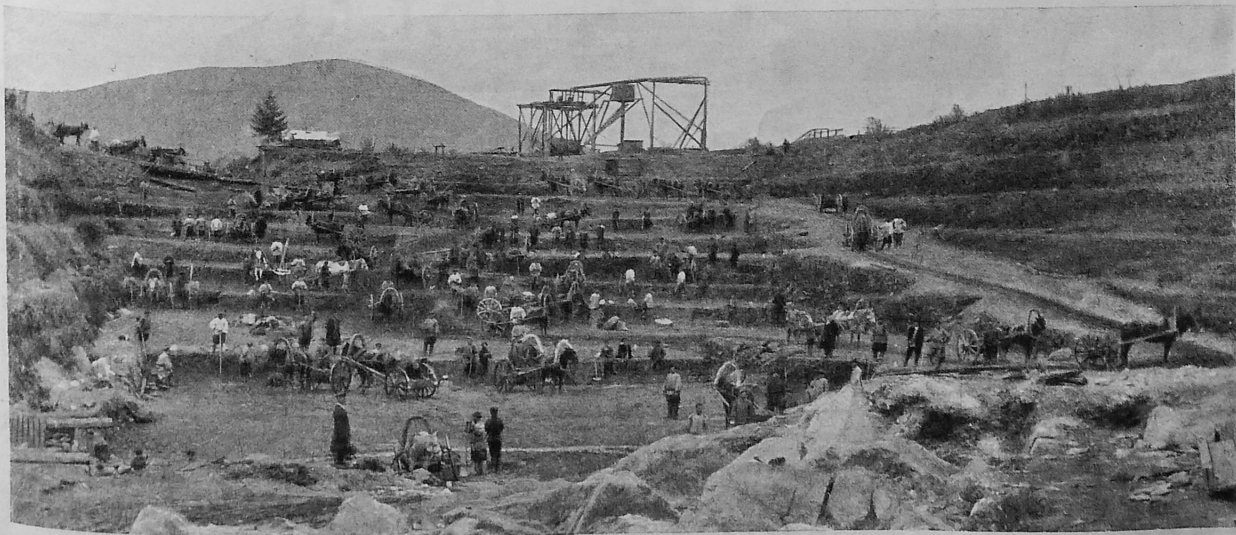
Открытый разръзъ. Добыча золотоносныхъ песковъ на промыслѣ Ленскаго товарищества.
