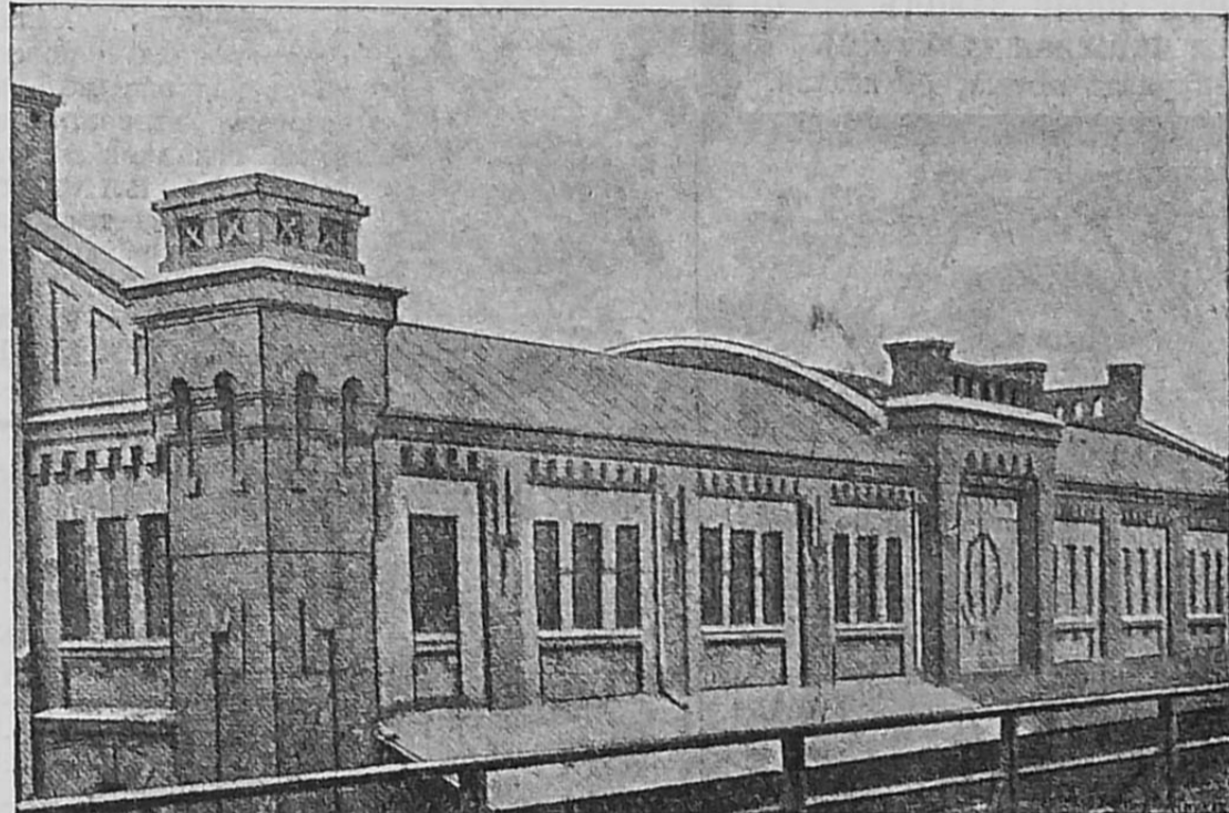
Крыша Сахарн. Склада пакгауза Ю.-З. ж. д., станция Одесса-Портъ, крытая Руберойдомъ.
