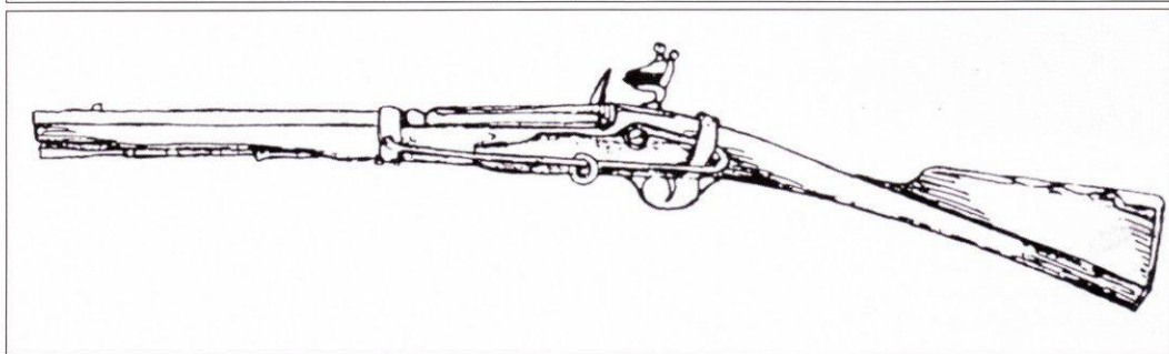
Огнестрельное оружие русской конницы: укороченный мушкет и карабин. Обе фузеи оснащены кремневым «французским замком». Русские драгуны широко использовали укороченные мушкеты. Они, безусловно, были длинны и неудобны, но зато обладали хорошей точностью и дальностью в стрельбе (рисунки с оригиналов в собрании Государственного исторического музея, Москва).
