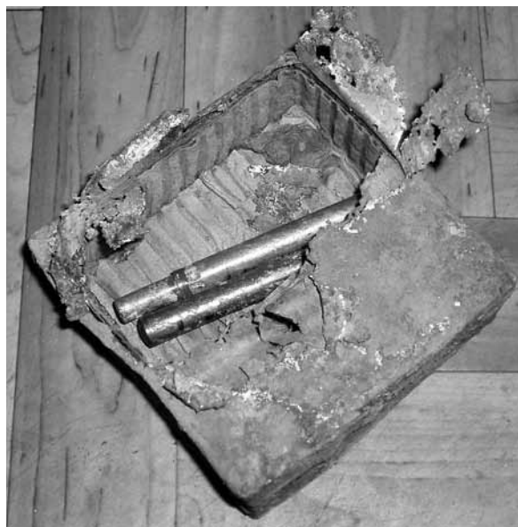
Рис. 4. Запалы в специальной укупорке
