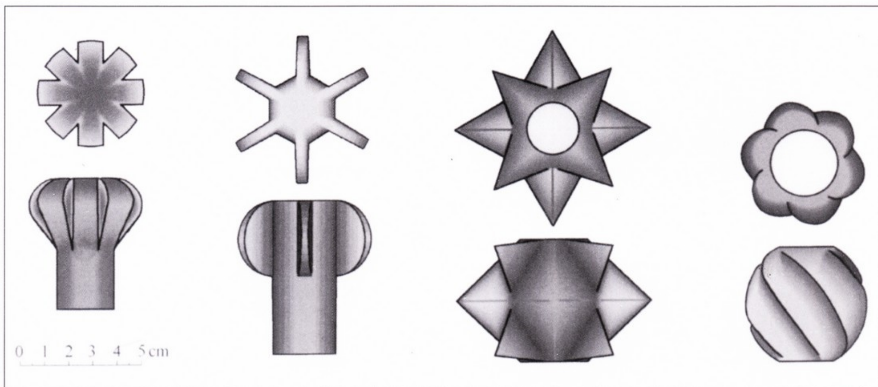
Византийские шестоперы. Все изображены в одном масштабе. Большинство головок железные, отдельные экземпляры бронзовые. Кроме представленных здесь встречались также шипастые шаровидные головки. Головки насаживались на деревянную рукоятку.
