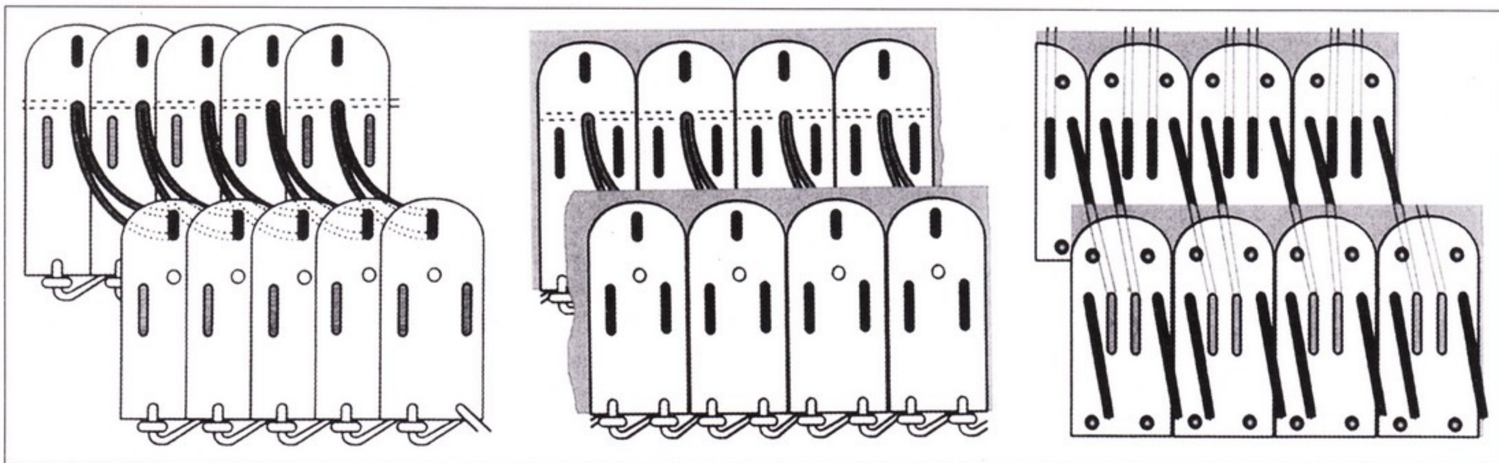
Слева: старая схема крепления пластинок ламелярного панциря. В позднее время она применялась только на конских доспехах. В центре: первый этап развития конструкции ламелярных доспехов в Византии. Пластинки пришнурованы к кожаному основанию, а не друг к другу. По соображениям ясности мы показали пластины с небольшим зазором между ними, но в действительности они пригонялись друг к другу как можно плотнее. Справа: последняя стадия эволюции византийского ламелярного панциря. Двойная шнуровка и парные заклепки надежно фиксируют пластинку. Слева виден край ткани. Для выравнивания кромки нечетные ряды завершались пластиками половинной ширины.
