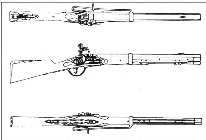
Гладкоствольный карабин образца 1787 года для гусар.
