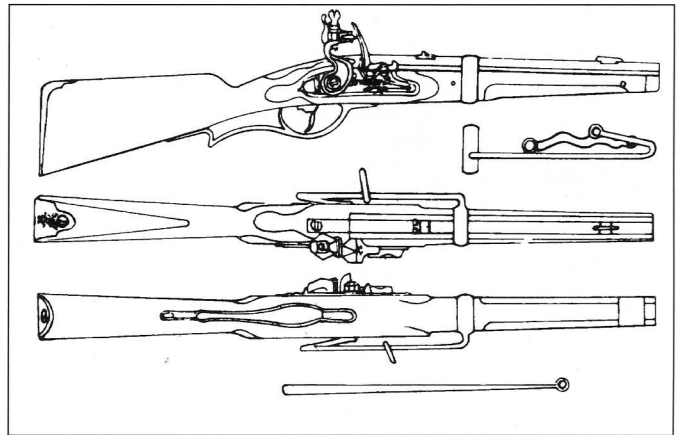
Нарезной гусарский карабин образца 1787 года. Обратите внимание на то, насколько гусарский карабин короче кирасирского и драгунского.
