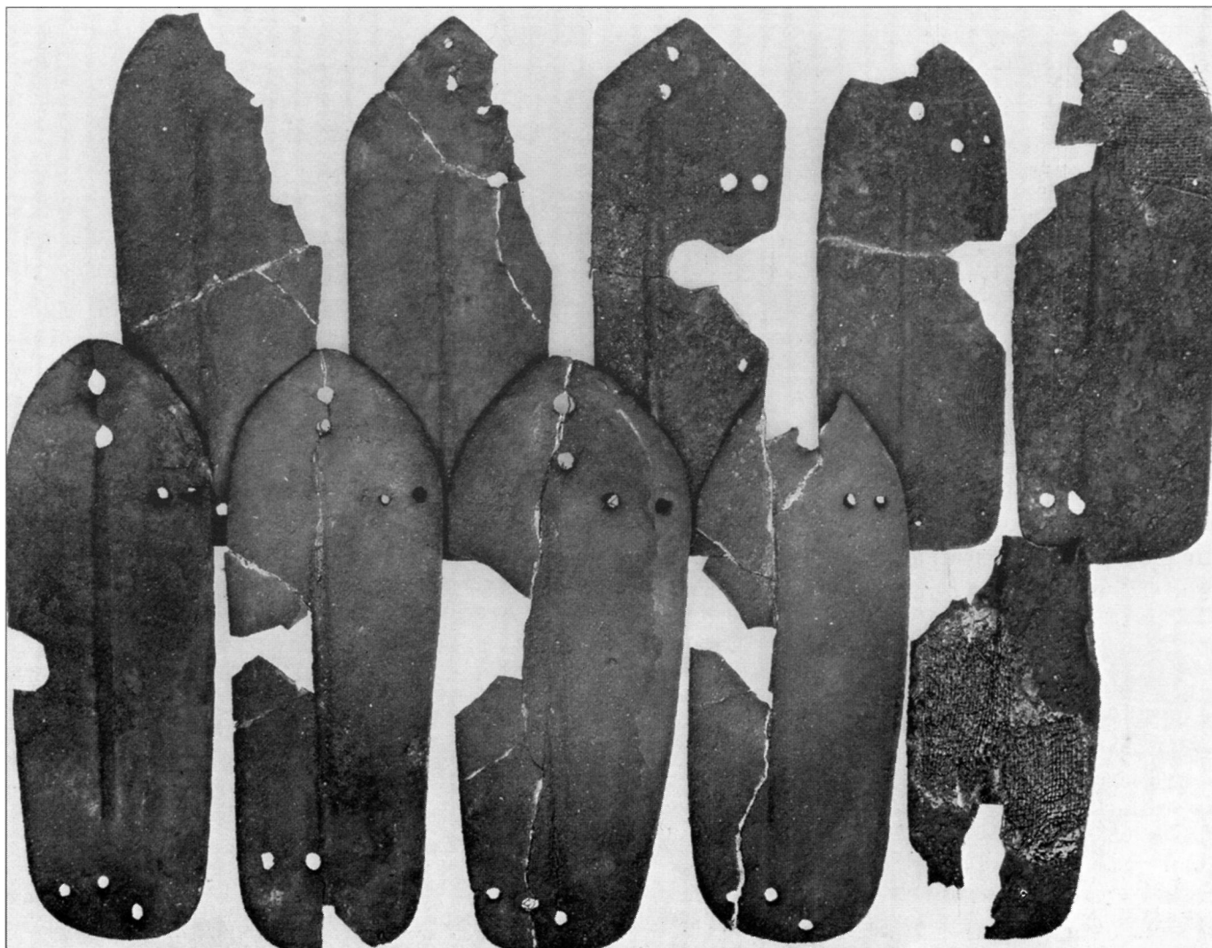
Бронзовая чешуя с доспехов XIV в. до Р.Х., найденная во дворце Аменхотепа III в Фивах. Отчетливо видны отверстия, через которые продевался шнур, крепящий чешую к кожаной или толстой матерчатой подкладке (остатки подкладки прилипли к левой верхней пластине). Гребень в центральной части пластины придавал ей большую механическую прочность, практически не сказываясь на массе. Изготовление чешуи требовало значительной технологической продвинутости. Доспехи были дороги, их могли позволить себе лишь наиболее богатые государства.
