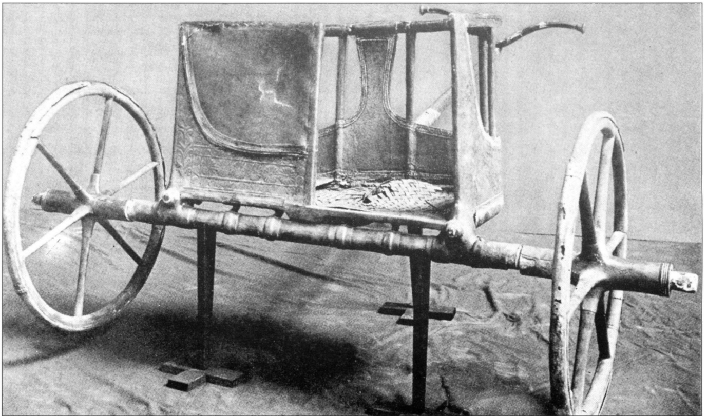
Колесница (1405-1370), вероятно, захваченная египтянами у хананеев. Обратите внимание на то, что ось проходит вдоль заднего края платформы, что улучшает маневренность и повышает скорость колесницы. Пол колесницы плетеный. Длинная ось с колеями 1,53 м повышает устойчивость колесницы на крутых поворотах.
