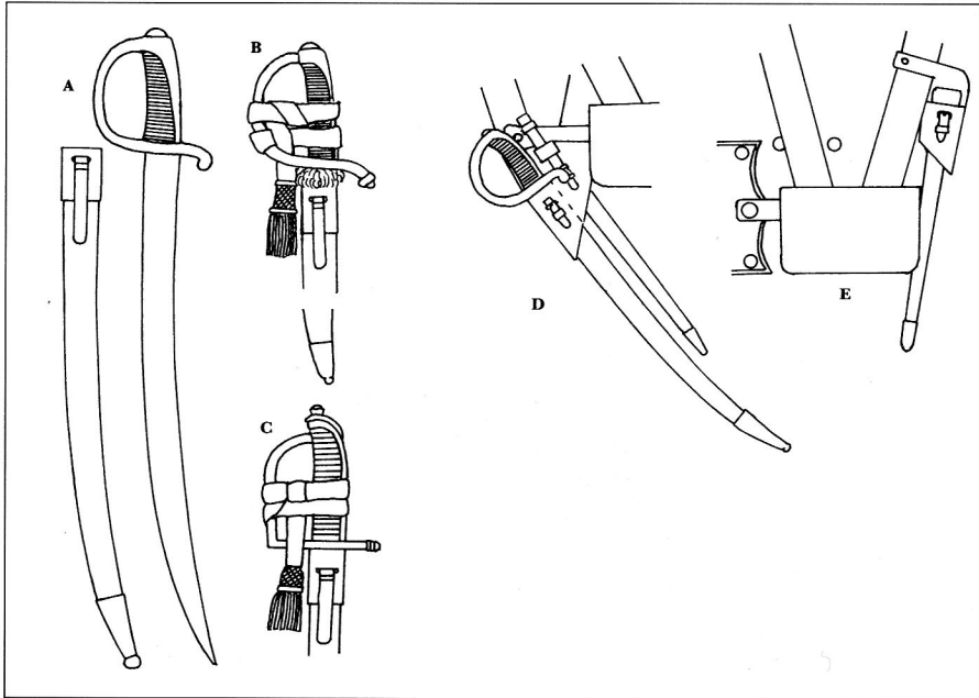
Сабля-брике: (A) An XI с латунной литой рукояткой. На рукоятке 28 поясков. (B) An XI с рукояткой с 32 поясками. Видны темляк и scavate (помпон между гардой и ножнами). (C) Сабля образца 1790 года, созданная на базе сабли образца 1767 года. Типичная угловатая гарда. Такие сабли состояли на вооружении легкой пехоты вплоть до 1804 года. Пехотная экипировка. (D) Сабля-брике и штык в комбинированных ножнах. (E) Штык, подвешенный на перевязи патронной сумки. Так штык носили в полках линейной, а позднее и легкой пехоты.
