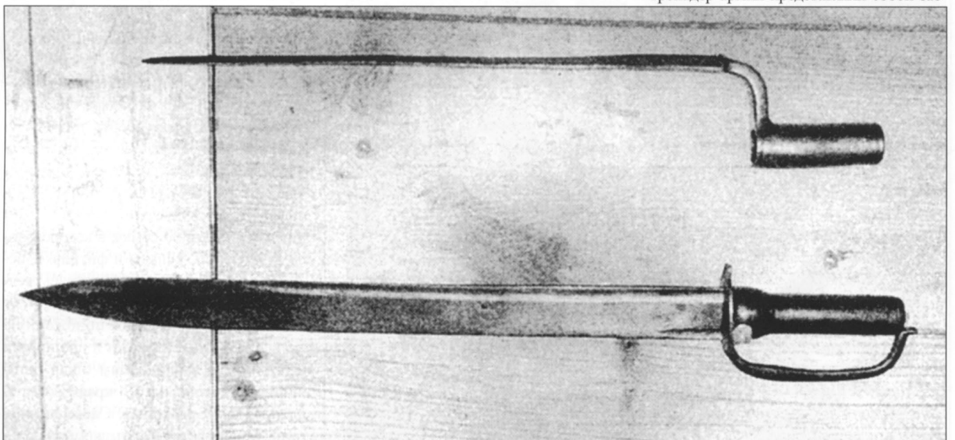
Штык и багинет русской армии, 1700-1725 годы. Первоначально русская пехота вооружалась багинетами, рукояти которых вставлялись в стволы фузей. Позже багинеты сменили штыки, которые можно было прижечь к стволу, не теряя возможности вести огонь.
