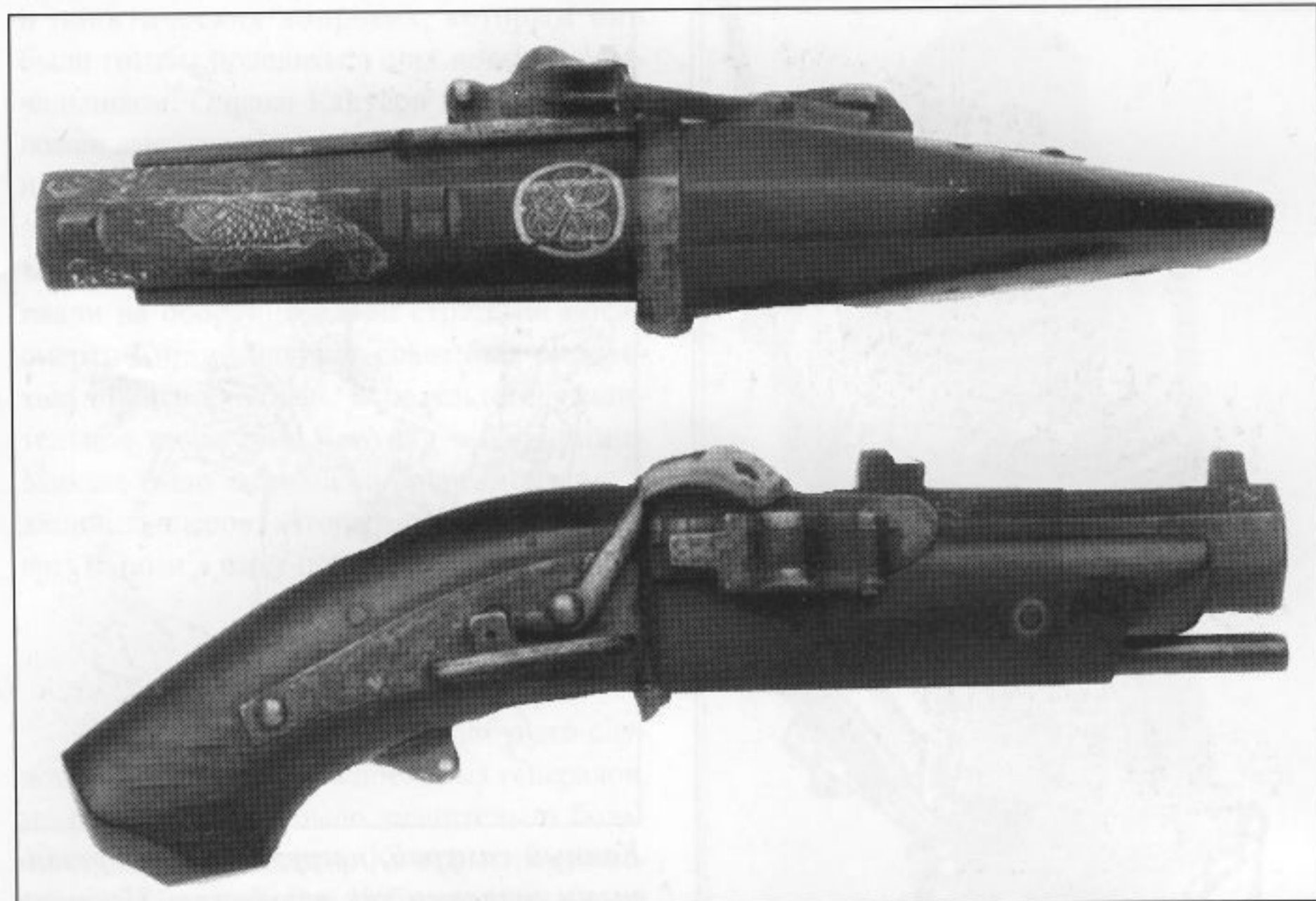
Фотографии с двух ракурсов миниатюрной аркебузы хорошо показывают детали фитильного замка. Запальное отверстие закрывает прикрепленная на петлях латунная крышка, которая предохраняет от преждевременного воспламенения. Тлеющий фитиль крепился на конце серпантина. Шомпол закреплен под стволом. На верхней стороне ствола этот экземпляр несет мон (символ) Токугава.
