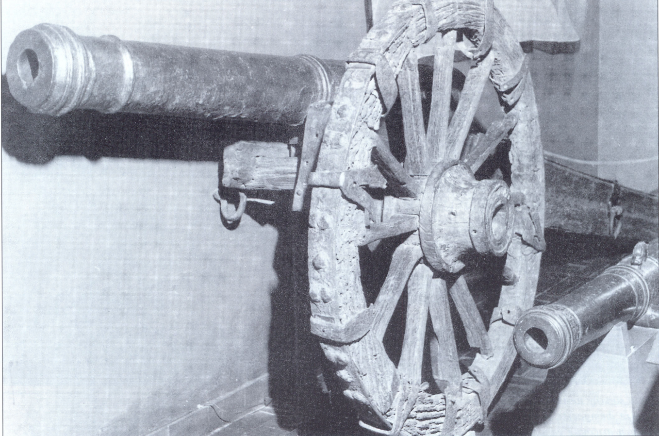
Пушка начала XVII в. с раздвижными станинами. Лафет обнаружен на дне Вислы под Варшавой в 1913 г. Размер колес позволяет предположить, что на лафете стоял шестифунтовая пушка со стволом длиной 27 калибров, так называемый Oktav-Kartaun. На лафет наложен подходящий по размеру ствол.
