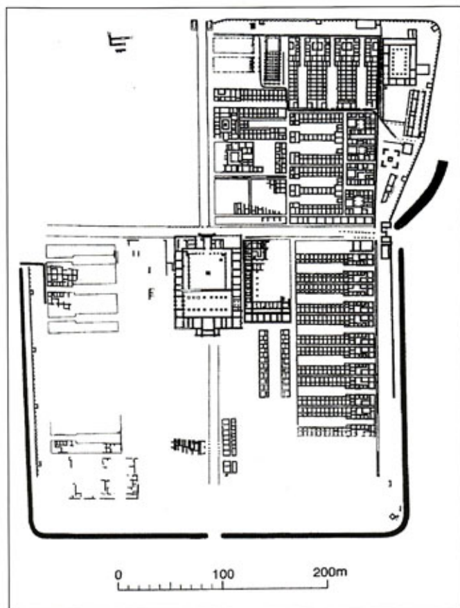
План крепости Новиомаг (Неймеген, Голландия). Крепость построена около 70 г. X Gemina на месте старой крепости, сооруженной еще во времена Августа. Перестройка крепости шла в несколько этапов. Полностью крепость перестроили в камне около 100 г.
