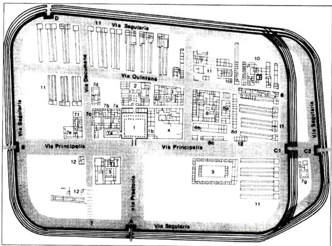
План августовской крепости Хальтерн, Германия. Первоначальная площадь крепости 16,7 га, позднее крепость расширена до 18 га. Указаны следующие постройки: Принципия (1), преторий (2), офицерские дома (7), мастерские (8), казармы (11), госпиталь (9). Главные ворота (porta praetoria) обозначены литерой А. Литера D обозначает задние ворота (porta decumana).
