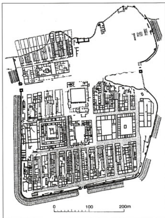
План крепости Карнунтум (Бад-Дойч-Альтенбург, Австрия), расположенной на Дунае на территории римской провинции Паннония. Раскопки здесь велись с конца XIX в. Различий по историческим слоям не делалось, данный план относится в основном к III в. н.э., когда здесь стоял XIV Gemina.
