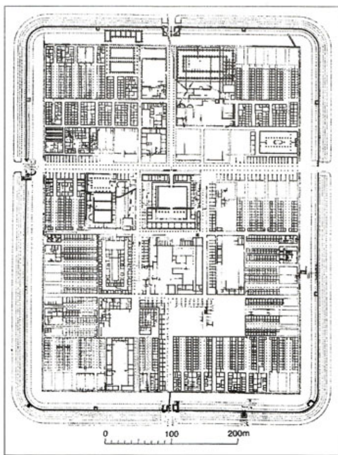
Крепость Новезиум (Нейсс, Германия) построена около 40 г. н.э. Позднее ее дважды перестраивали в камне. В 70–100 гг. крепость занимал VI Victrix. На плане указаны фундаменты зданий, возведенных в ходе обеих перестроек.
