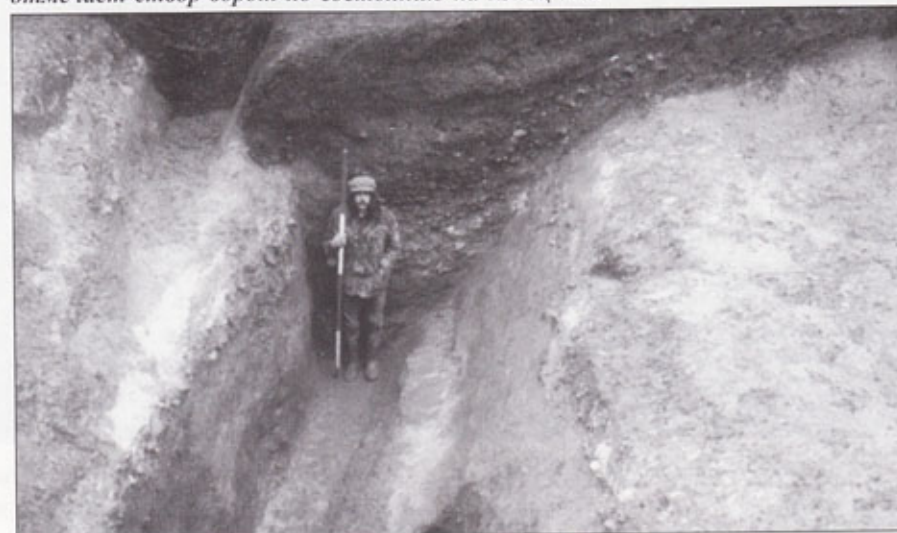
Раскопки, проведенные в конце 1970-х гг. обнаружили угол крепости Эксетер. Глиняный вал шириной 6 м уцелел на высоту 0,9 м. Примерно в 8 метрах перед валом проходит ров глубиной 3,8 м и шириной 4,2 м.
