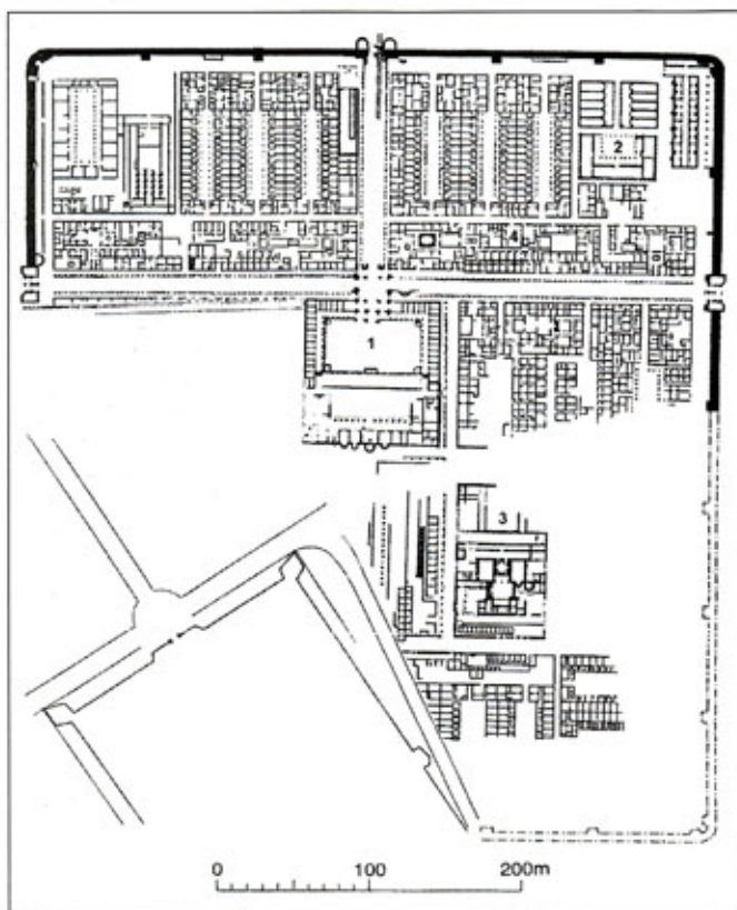
План крепости Ламбезис (Ламбез, Алжир), основанной III Augusta при Адриане и перестроенной в 250-х гг. Французы в конце XIX в. построили юго-западной части крепости тюрьму, которая закрыла античные фундаменты. Цифрами обозначены: (3) бани, (4) квартал трибунов, (2) мастерские.
