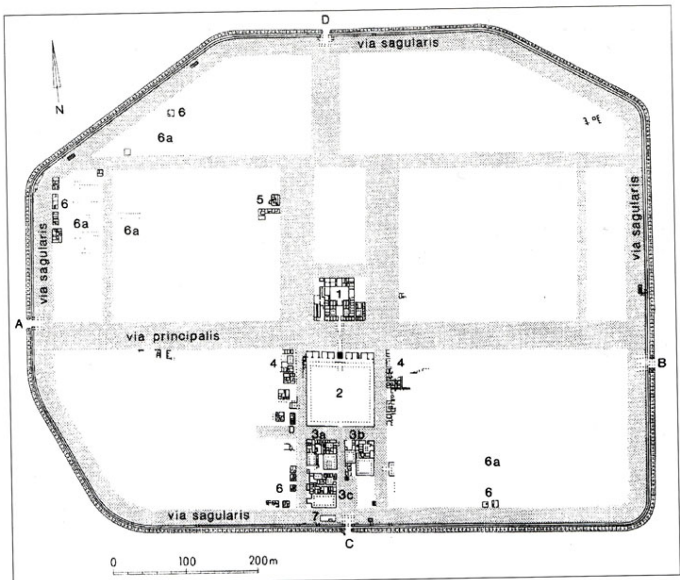
План крепости Обераден (Германия). Площадь крепости 56 га, она датируется периодом кампаний Друза за Рейном (11–9 гг. до н.э.). Это самая старая из известных крепостей. Выделены следующие постройки: преторий (1), принцепия (2), дома офицеров (3), дома центурионов (6), казармы (6a). Литерой С отмечены porta praetoria.
