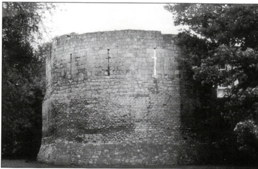
Так называемая Многоугольная башня в Йорке (Англия) возведена около 300 г. в западном углу крепости Эбуракум. На юго-западе протекает река Ус. Особая архитектура башни, по-видимому, должна была производить впечатление на простолудинов, плавающих по реке.
