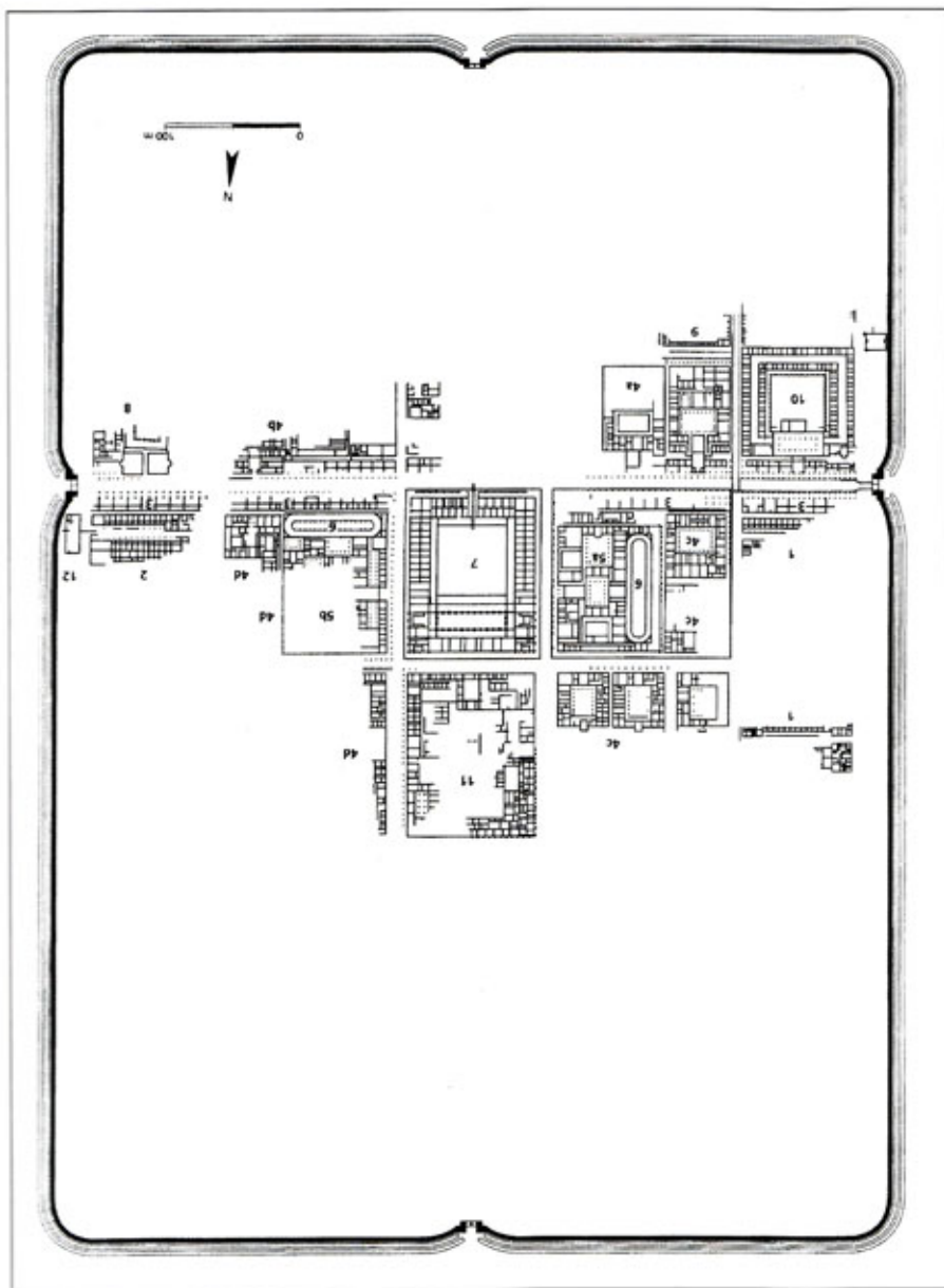
Значительная площадь крепости Ветера остается не раскопанной. Западную половину крепости занимал V Alaudae, а восточную XV Primigenia. Обозначены: казармы (1 и 2), дома трибунов (4c и 4d), две претории (5a и 5b), госпиталь V Alaudae (10), центральная принцепия (7).
