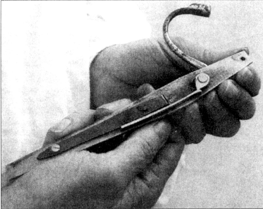
Конструкция фитильного замка. Замок действовал следующим образом. Когда стрелок нажимал на кнопку, соединенную со спусковым рычагом, последний отпускал серпентин, который падал на затравочную полку.
