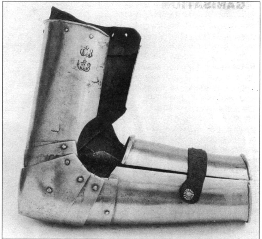
Левый вомбрас из Глазго, фрагмент итальянских доспехов. Налокотник частично разобран, видно устройство гибкого сочленения. На верхней части вомбраса заметны клейма мастера.
