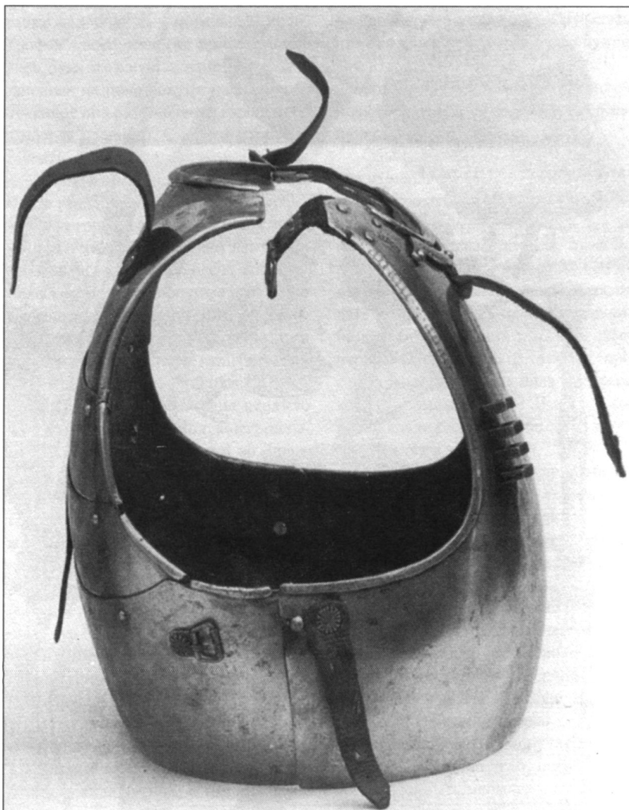
Кираса, вид справа. Видны крепления упора для копья на грудной пластине.
