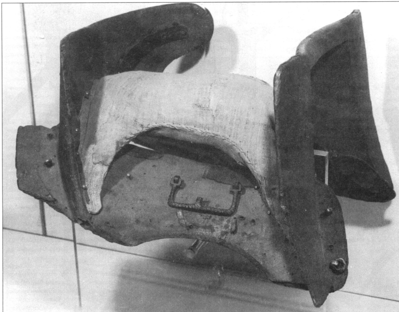
Боевое седло из могилы Генриха V. Холщовое сиденье, набитое сеном имеет высоту 12 см. Холст приклеен ко всем деревянным поверхностям. Чехол из голубого бархата с лилиями утерян. Прямоугольное кольцо над остатками двойной подпруги служит для подвески стремени. Кольца на луках седла служат для крепления ремней упряжи.
