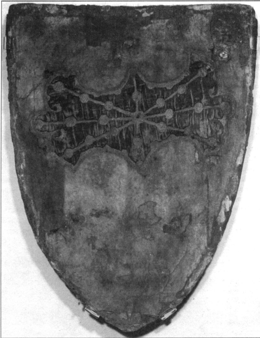
Внутренняя сторона дубового щита, подвешенного над могилой Генриха V. Щит имеет амортизатор из трех слоев холстины с проложенным между ними конским волосом. Снаружи щит отделан парчой и украшен изображением плюща и лилий. Упор для руки из малинового бархата с гербом Наварры (откуда родом жена Генриха). Наружная сторона щита обшита в четыре слоя холстом и раскрашена.
