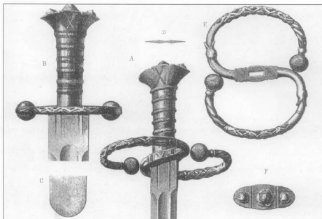
Ландскнехтский катцбальгер. Katz — немецки — кошка, balgen — драгься. Так что слово «катцбальгер» можно перевести как «оружие для кошачьей драки». А и В. Рукоятка, украшенная изображением андреевского креста. С. Кончик клинка. D. Поперечное сечение клинка. E. S-образное перекрестье. F. Головка эфеса, вид сверху.
