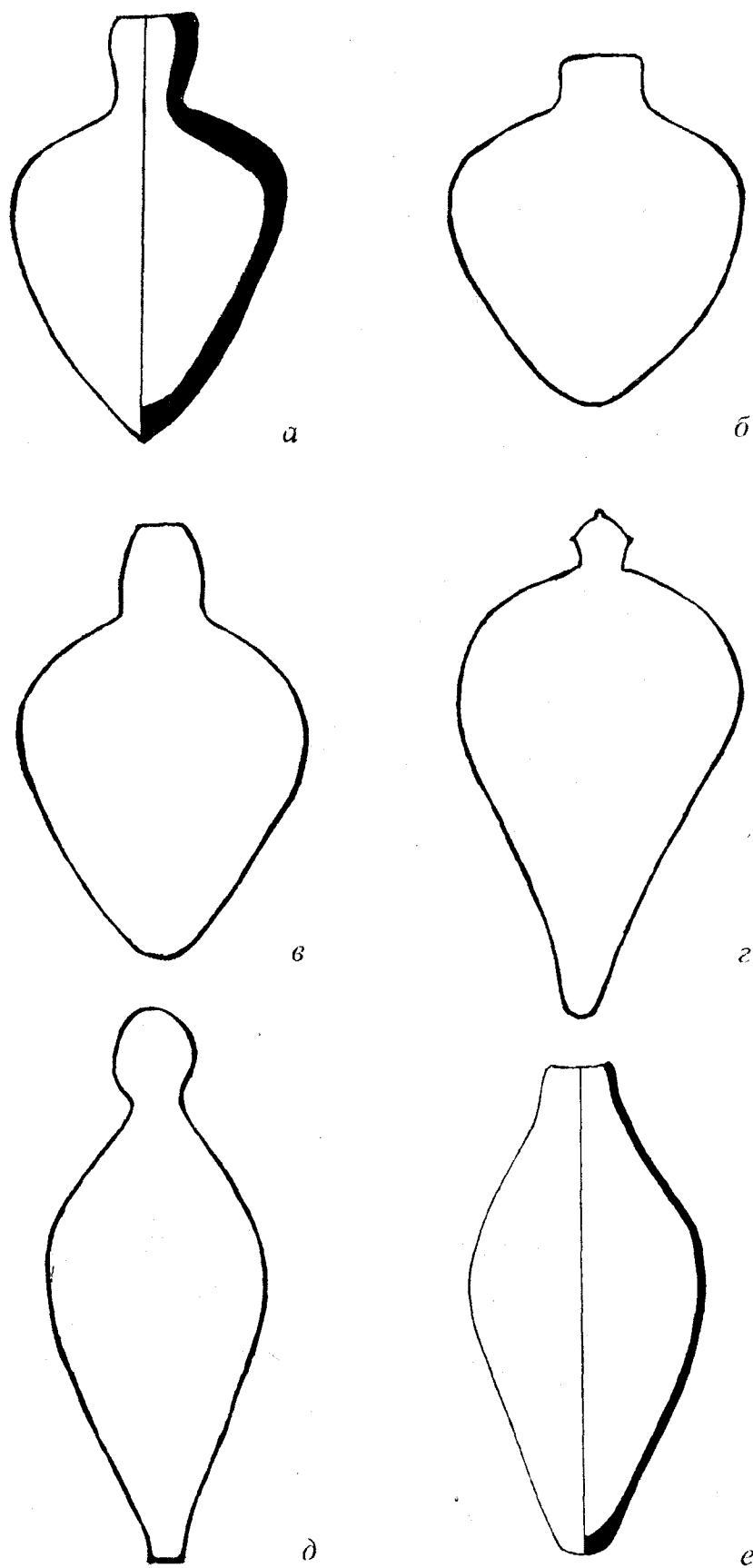
Рис. 4. Формы стеклянных сфероконов: а – Афрасиаб XI–XII вв.; б – Биляр, кон. XII – нач. XIII в.; Египет или Сирия, кон. XIII в.; г – Средняя Азия, XIII–XIV вв.; д – Царевское городище, XIV в.; е – Теке-джир, XIV в.
