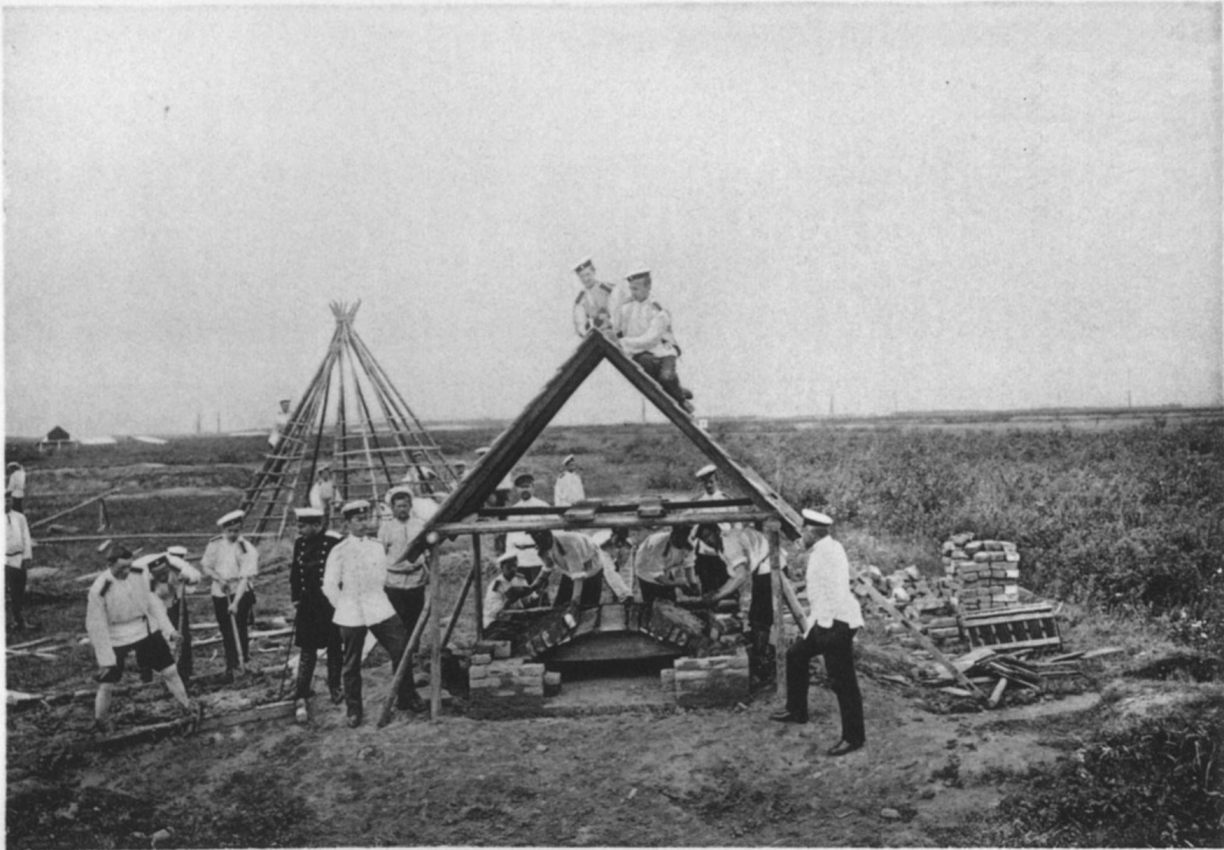
Бивачная работы (печь).
