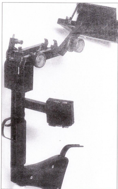
Практическое применение устройства для ведения огня из укрытия (Deckungziehlgeraet, Dezetgeraet).
