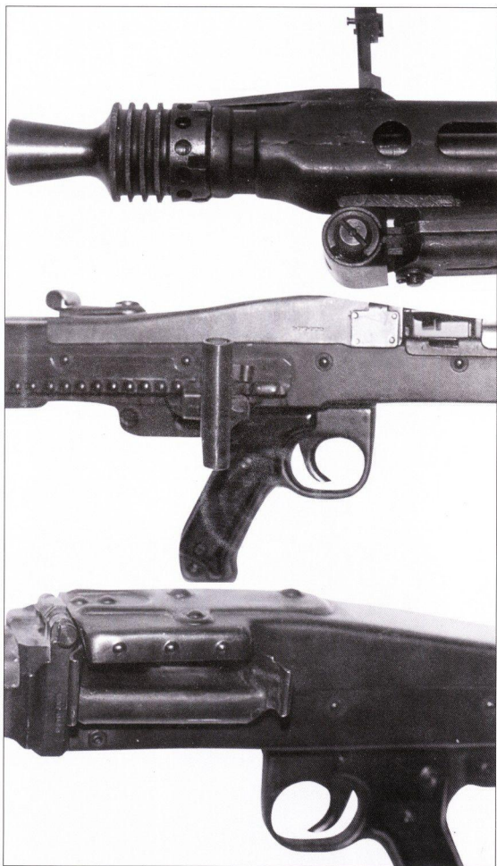
Пулемет MG 42 раннего выпуска, сошки (Zweibein) сняты. Обратите внимание на характерную форму рукоятки затвора.
