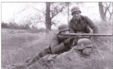
Французский пулемет Mitrailleuse de 7,5 mm mle 1931 (Reibel) . На вооружении немецкой армии этот пулемет известен как 7,5 мм Katpfwagen-MG 311(f) . Это французский танковый пулемет, оснащаемый 150-зарядным барабанным магазином. Немцы добавили к пулемету приклад и сошки, превратив его в пехотный пулемет. Снимок сделан военно-технической службой США.
