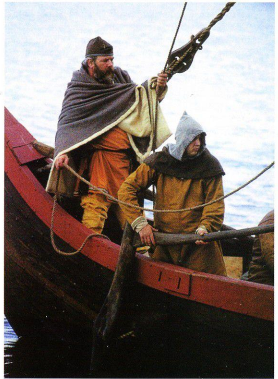
Установленное на правом борту рулевое перо закреплено на доске верхнего яруса обшивки. Горизонтальным румбелем управляет команда, находясь в корме. Благодаря этому в больших размерах корабль развивал скорость до 10 км/ч.
