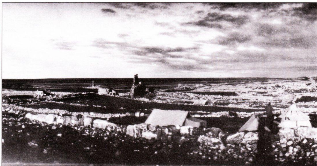
Южный затвор илюза в Даре, вид изнутри города. Видны два этапа строительства стены. На первом этапе при Афанасии стену возвели на высоту 10 м. Верхняя, более тонкая часть стены пристроена при Юстиниане.
