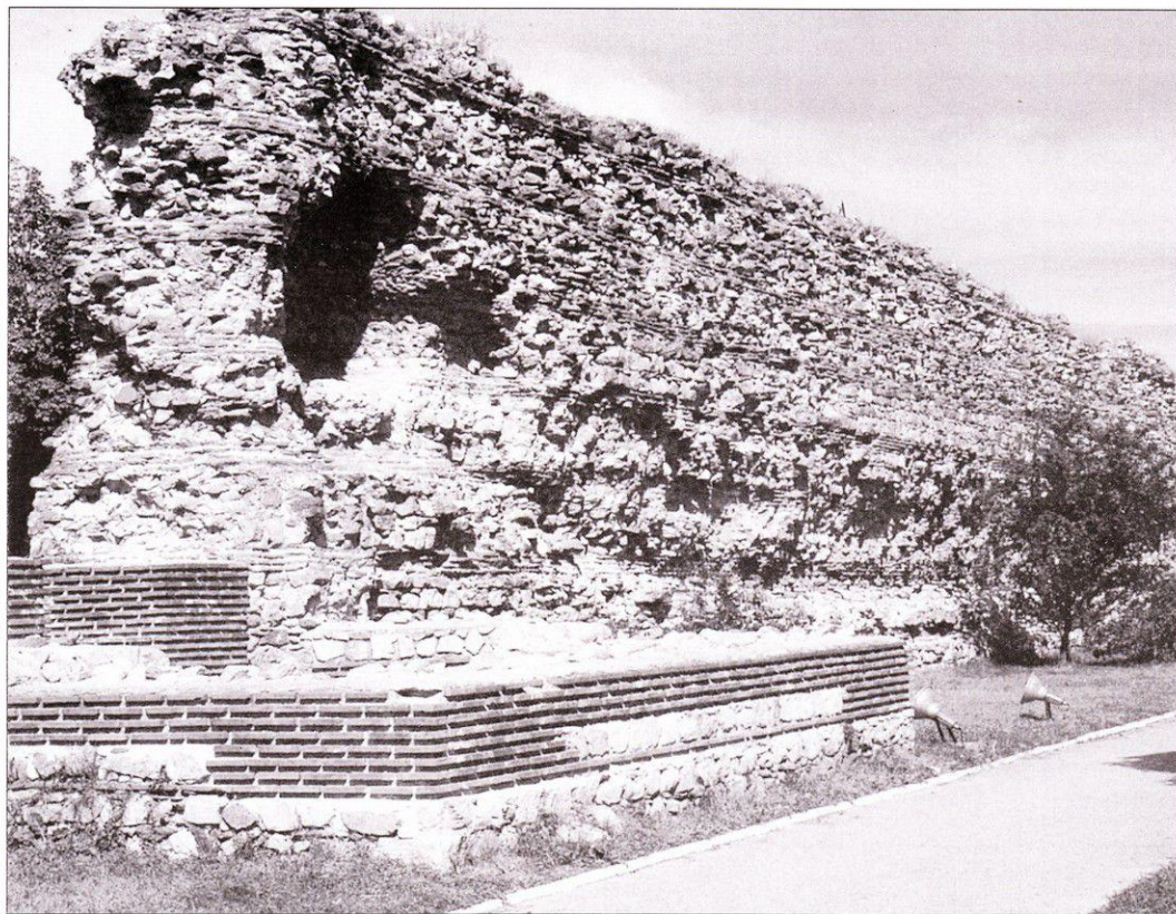
Укрепления Диоклетианополиса (Хиссар, Болгария). Характерная для римских укреплений кладка из двух слоев кирпича, между которыми слой булыжника.
