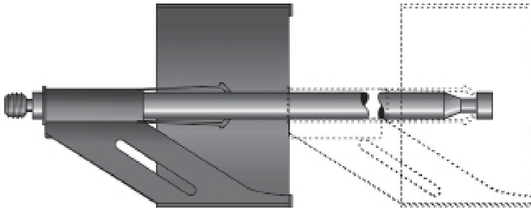
Перемещение стабилизатора после выстрела Рис. Е. Кравченко
