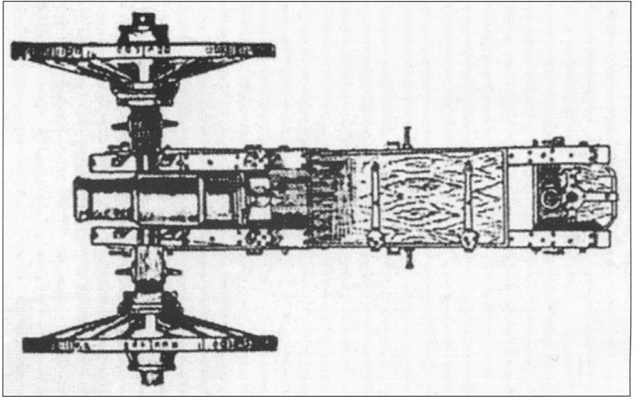
Вид сверху на полупудовый (20-фунтовый) единорог. Его компактная конструкция включала небольшой зарядный ящик, встроенный в хобот лафета. Это позволяло орудию действовать без сопровождения зарядного ящика, необходимого для полковой 3-фунтовой пушки.
