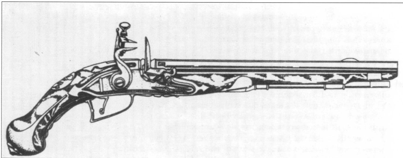
Русский кавалерийский пистолет образца 1735 г. Это стандартный кавалерийский пистолет, находившийся на вооружении русской армии с 1735 по 1766 г. Рисунок выполнен по образцу, изготовленному в Туле, из коллекции Государственного Исторического музея в Москве.
