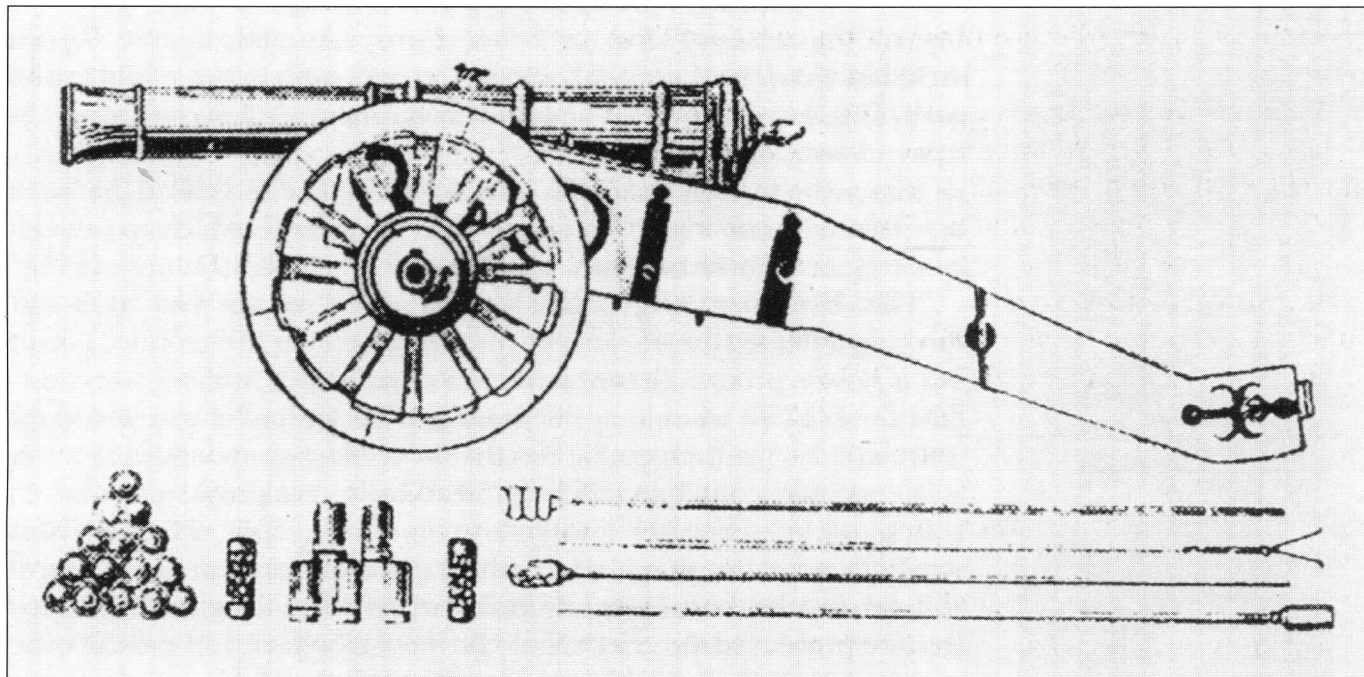
24-фунтовая пушка, одна из основных пушек колонны осадной артиллерии русской армии. Здесь же изображены инструменты (прибойник, банник) и различные выстрелы.
