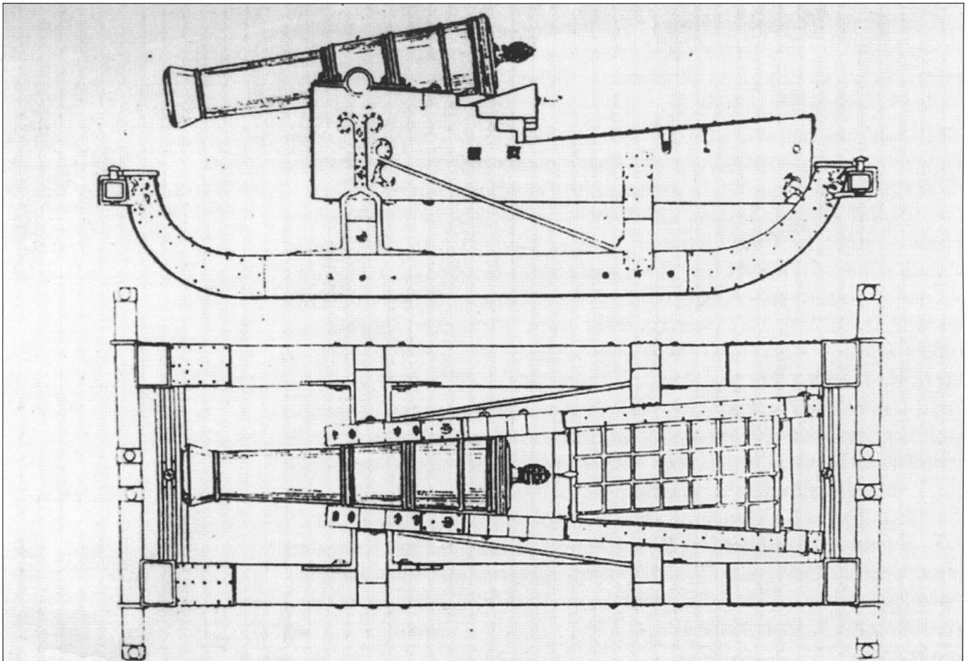
Модификация 3-фунтовой пушки, произведенная зимой 1757/58 гг. в Восточной Пруссии. Лафет установили на санное полозья. Для буксировки такой пушки использовали модифицированной упряжь.
