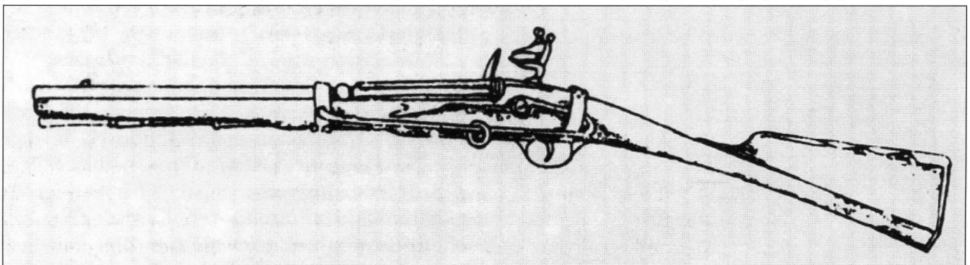
Русский кирасирский карабин (1735-1765). В русской кавалерии карабинами вооружались только кирасиры. Обратите внимание на подвеску карабина к перевязи. Перевязь крепилась к кольцу, свободно скользящему по прутку. Подвешенный карабин опускался дулом вниз. Рисунок экспоната из Государственного Исторического музея в Москве.
