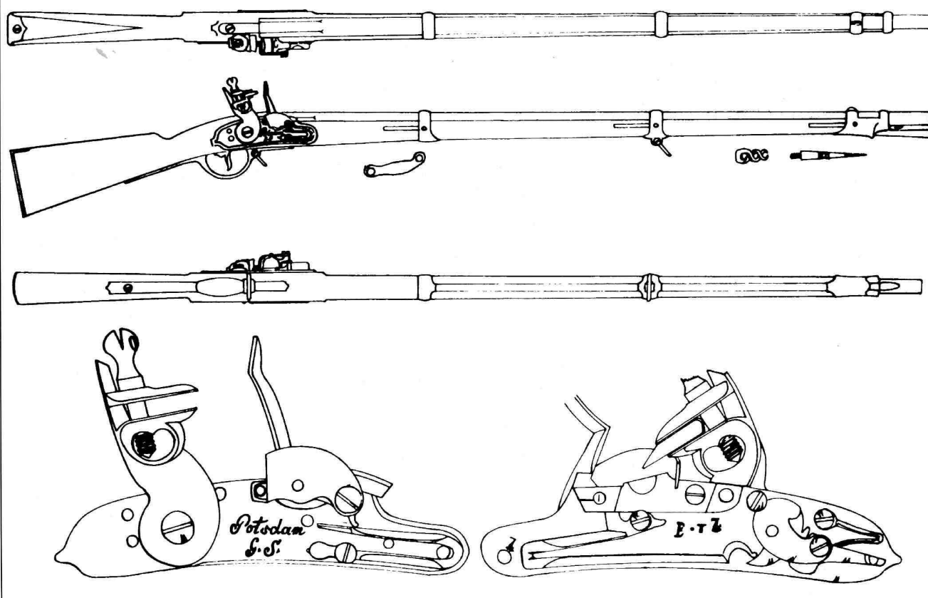
Рисунок общего вида мушкета образца 1809. Общая длина 143 см, длина ствола 104 см.
