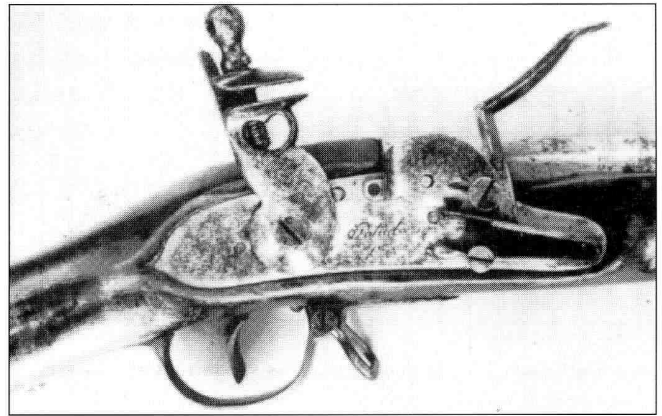
Замок мушкета образца 1809, изготовленного в Потсдаме.
