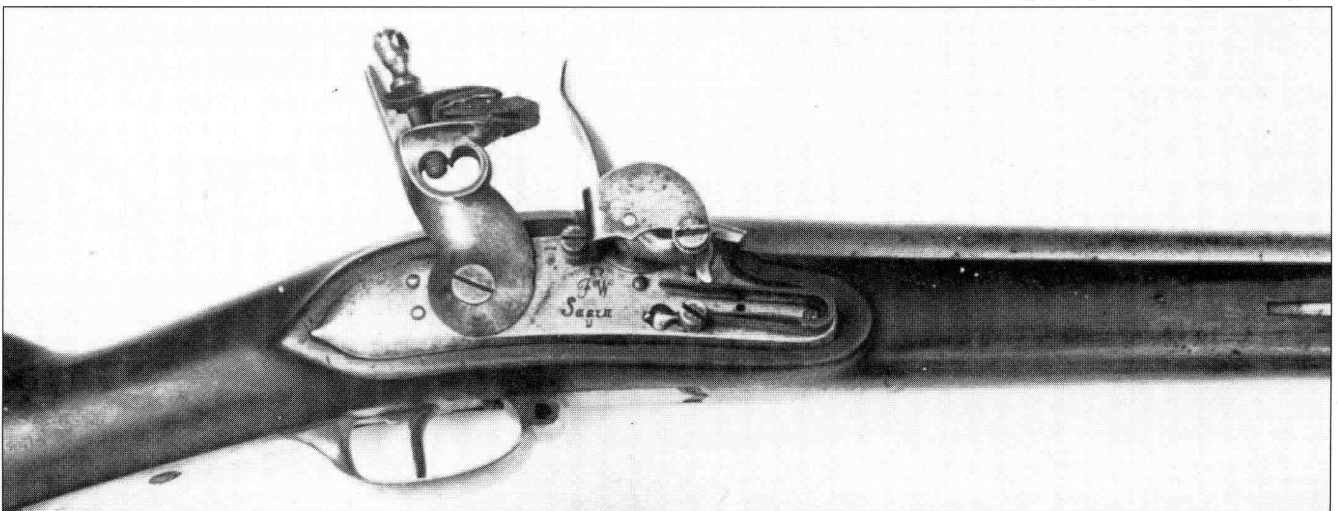
Замок мушкета образца 1809, изготовленного в Саарне, Рейнланд.
