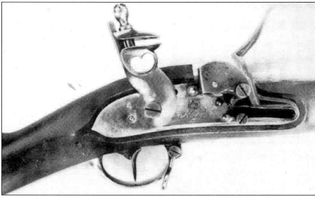
Замок «нового» прусского мушкета образца 1809, изготовленного в Нейссе в Верхней Силезии. Обратите внимание на щиток вокруг полки, защищающий затравку от непогоды, а лицо стреляющего от вспышки затравки.
