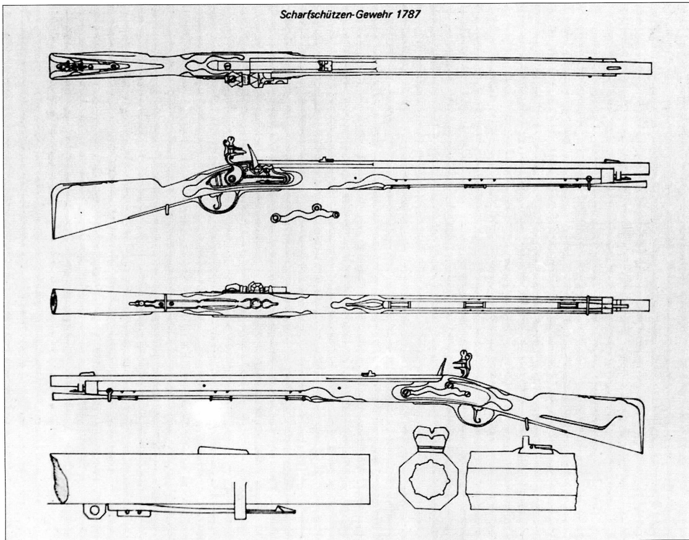
Снайперское ружье образца 1787 года. Длина 124 см, калибр 18,5 мм. Всего было изготовлено около 10000 таких ружей, которые использовались в стрелковых отделениях линейных и легких пехотных батальонов. Крупным планом показано пружинное крепление штыка, нарезка ствола и регулируемый целик.
