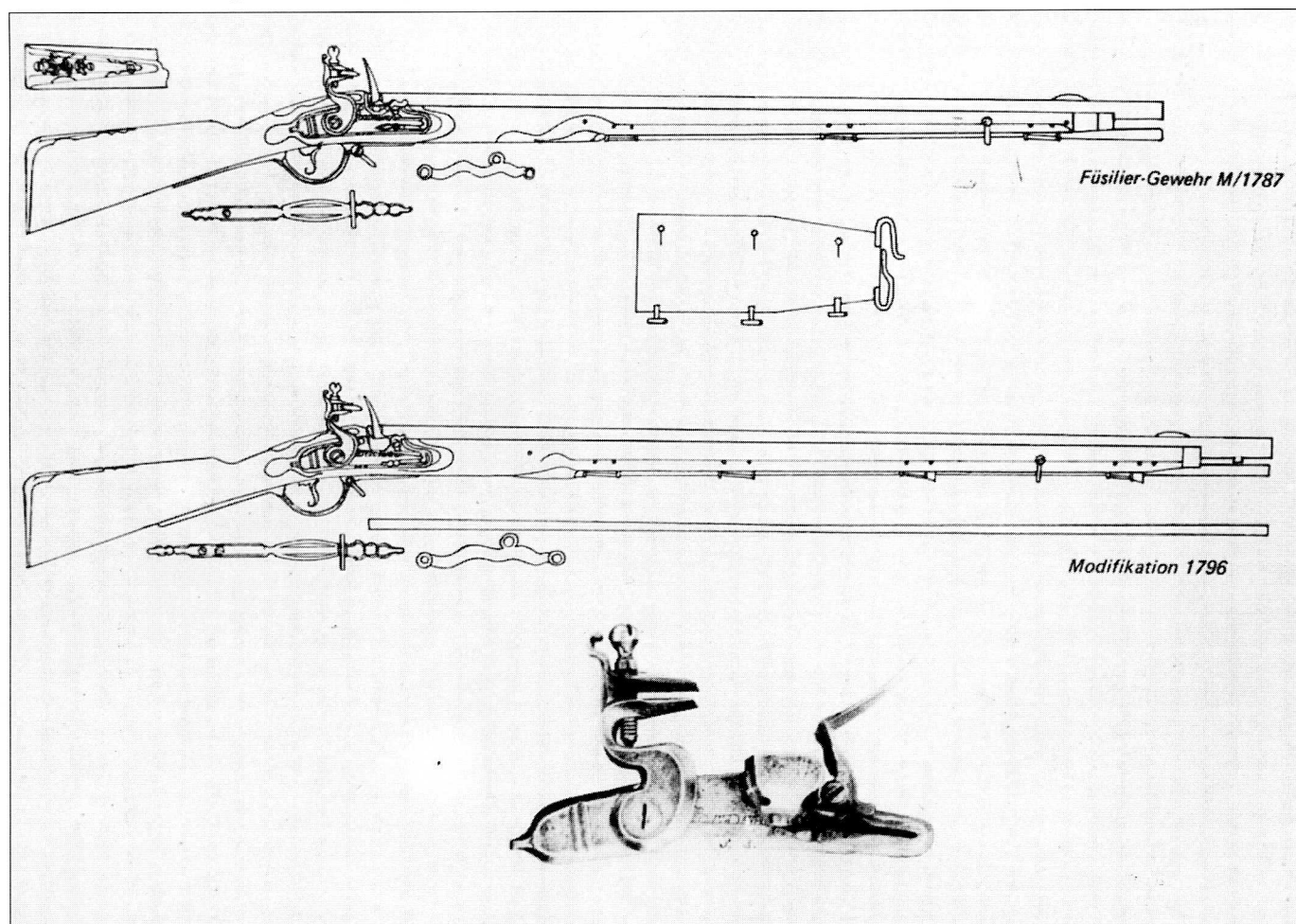
Фузилерский мушкет: (вверху) мушкет образца 1787 года. Длина 134 см, ствол 95 см, калибр 18 мм, внизу изображен кожаный чехол на замок. Внизу: модификация мушкета 1796 года. Длина 145 см, ствол 104 см. Для своего времени мушкет был очень продвинутым оружием. На фотоврезке внизу показан замок с щитком, защищавшим затравку от ветра и дождя, а также гасящий выброс при выстреле.
