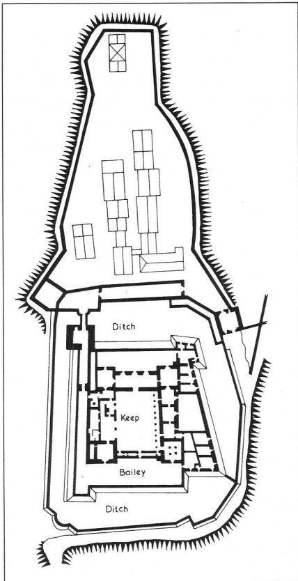
План замка Торрекиара. Похожий план имели Мантуя и Феррара. Но наружное устройство Торрекиары совершенно иное. Замок был построен Пьером-Марией Росси в 1448-1460 годах в провинции Парма.
