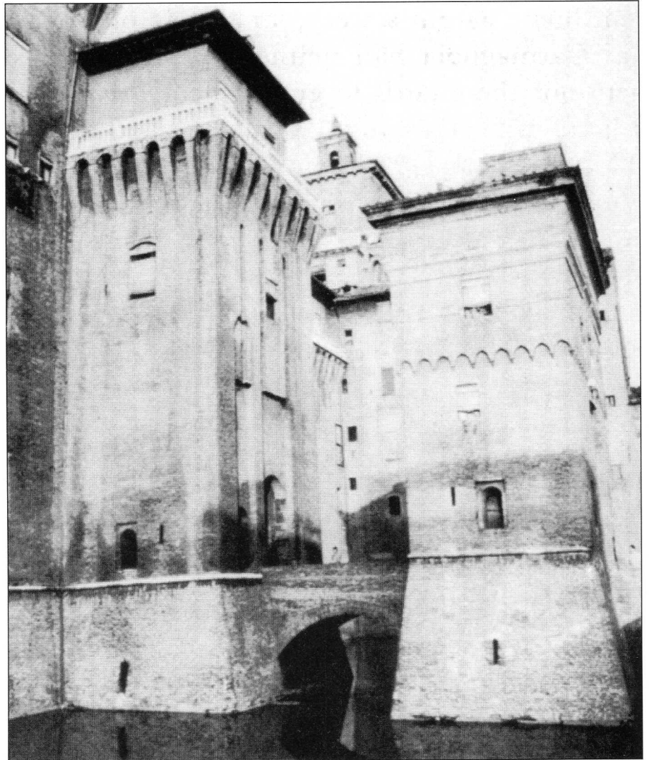
Замок Кастелло-Эстенсе в центре Феррары был построен в 1383 году. Замок построен на равнине. План замка регулярный с угловыми башнями и заполненным водой рвом. Использование кирпича, а не камня - отличительная особенность замков, возведенных в долине реки По.
