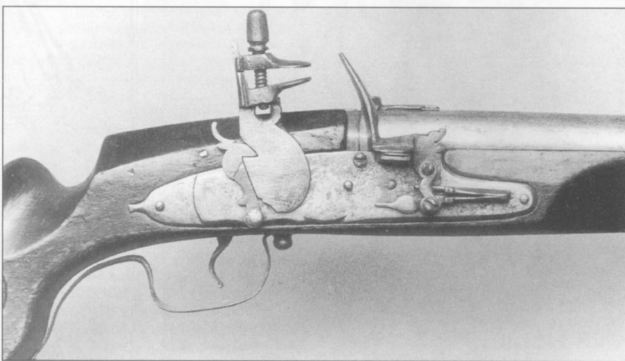
Кремниевые замки. Кремневыми мушкетерами вооружались солдаты, охранявшие артиллерийские орудия, так как тлеющие фитили представляли собой опасность вблизи больших складов пороха. Несколько отдельных рот королевской пехоты также вооружались кремневыми мушкетерами. Здесь показаны два наиболее распространенных типа замка: голландский замок (вверху) и французский замок (внизу).
