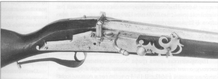
Фитильный замок. Перед выстрелом мушкетер должен был убедиться, что фитиль попадет в центр затравочной полки. При выстреле открывалась крышка полки, и фитиль поджигал затравочный порох.
