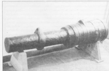
Различия в форме ствола и пороховой камеры этого венгерского орудия XV века из мягкой стали и предыдущего образца вполне очевидны.
