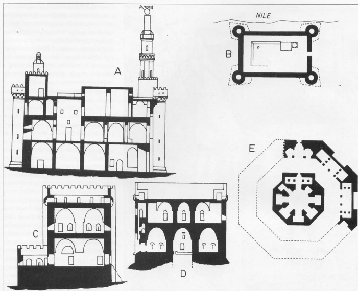
А. Разрез через центральные помещения и мечеть замка Кайт-бея, контролировавшего александрийскую гавань, 1479 г. В. План небольшого форта Кайт-бея, контролирующего северный рукав Нила у Рашида, 1479 г. С. Восстановленный разрез через «Устевую башню», Триполи, Ливан, около 1475 г. Бастион слева пристроен в XVII–XVIII вв. D. Разрез через «Львиную башню», Триполи, Ливан, около 1475 г. E. План Калат-аль-Тина, Синай, построенного в период правления султана аль-Гури, начало XVI в.
