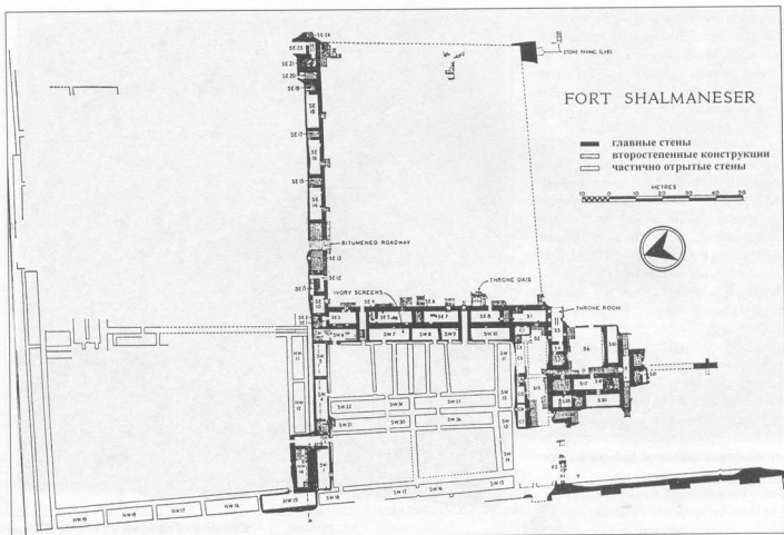
План арсенала «кал машарту», построенного Салманасаром III в Калху. Здесь имеется большой плац, королевские покои, склады для хранения провианта, оружия и трофеев. Клинописный список свидетельствует о распределении пленных: «командующему гарнизонного отряда боевых колесниц», «касситским и ассирийским пращникам». Подобного рода здания возводились в разных городах империи и служили базами для ассирийской армии.
