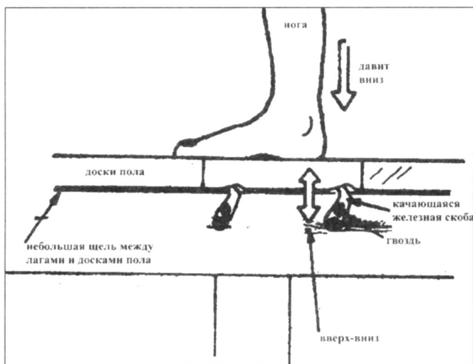
Принцип действия поющих половиц, замок Нидзё в Киото. Вопреки устоявшемуся мнению, скрип производит не сама половица, а металлические детали, которые обиваются друг относительно друга при надавливании на половицу.
