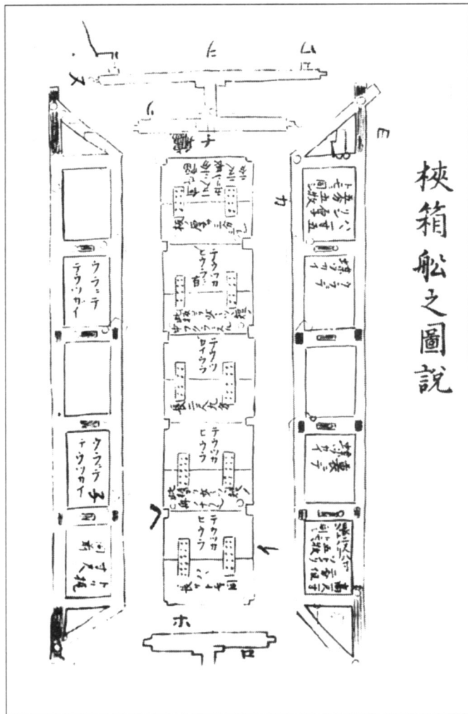
Складная лодка ниндзя, иллюстрация из «Бансен Сюкай». Детали соединяются между собой зажимами и обтягиваются водонепроницаемой тканью.
