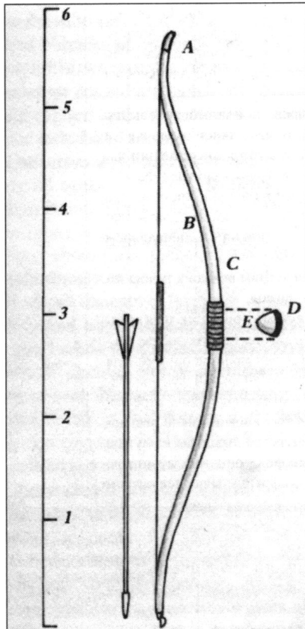
Конструкция длинного лука. А – законцовка лука, «нок»; В – «живот», «белли»; С – «спина» лука, «бэк»; D – заболонь; E – твердая древесина. Стандартная длина заготовки около шести футов.
