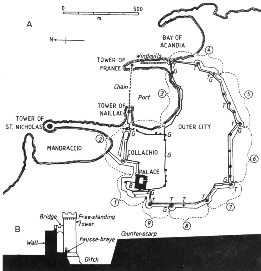
Фортификации Родоса, 1480 год. Г. Ворота, В. Главный бастион, Т. Башня. Участки стены. 1. Дворец магистра. 2. Французский. 3. Кастильский. 4. Итальянский. 5. Прованский. 6. Арагонский. 7. Английский. 8. Оверньский. 9. Германский. В. Разрез через сухопутную стену, 1480 год.
