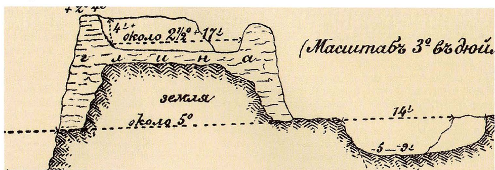
Профиль главной стены крепости Денгиль-Тепе. Литография 1889 г.
