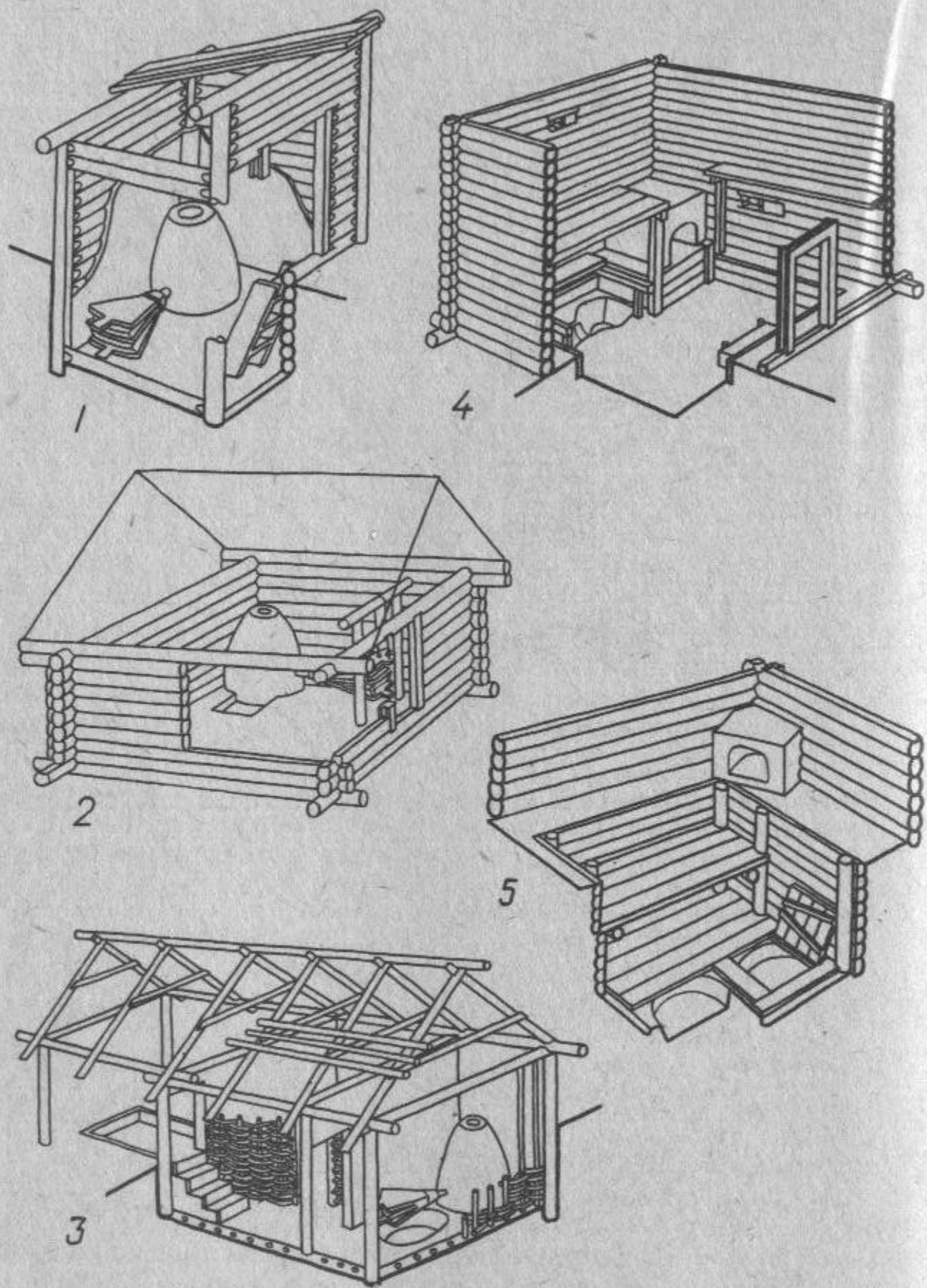
Ремесленные мастерские, открытые в Рязани: 1—3 — мастерские с домницами, где добывали железо из руды; 4 — мастерская костореза; 5 — мастерская для отливки бронзовых украшений. Реконструкции
