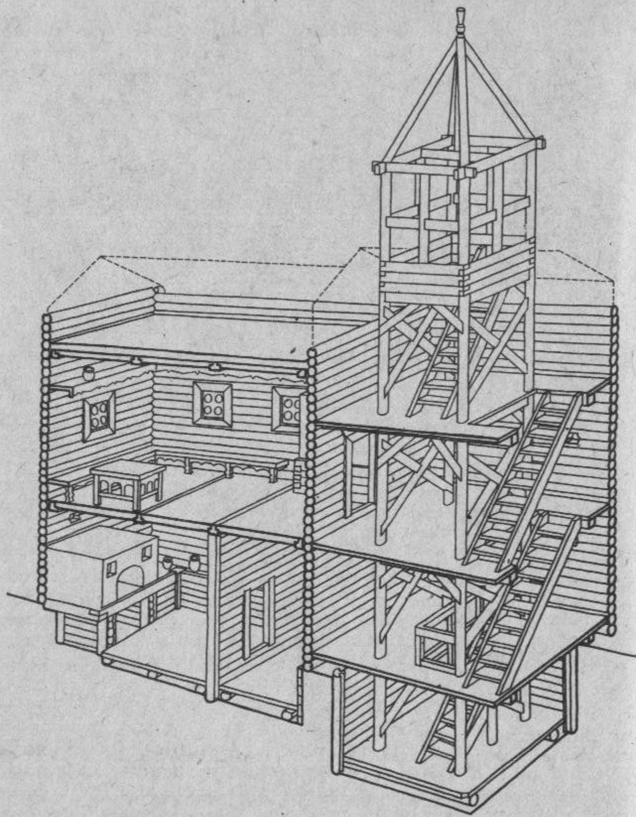
Реконструкция интерьера терема с башней-вежей. Здание воссоздано по расположению ям от несущих столбов, рассчитанных на высотную конструкцию, разному уровню полов в нижнем этаже, кирпичам от упавшей печи, находившейся в горнице. В помещениях терема показана меблировка — лавки, полки, столы: плотники называли это «нарядить нутро»
