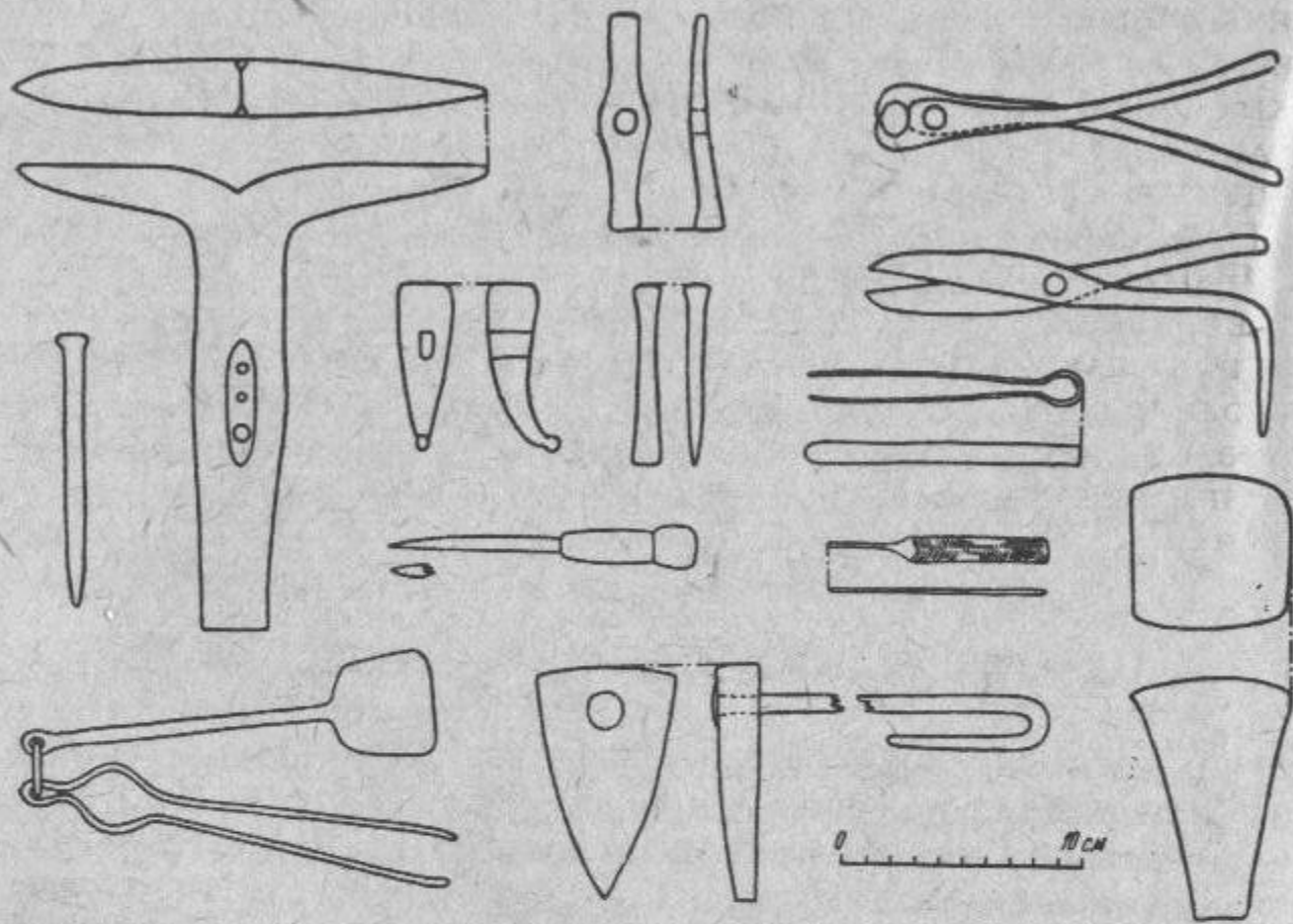
Ювелирные инструменты: фигурная наковальня, молотки, клещи-кусачки, ножницы по металлу, зубила, резец по металлу, напильник, пинцеты, паяльник, наковальня. Из книги: Колчин Б. А. Черная металлургия и металлообработка...
