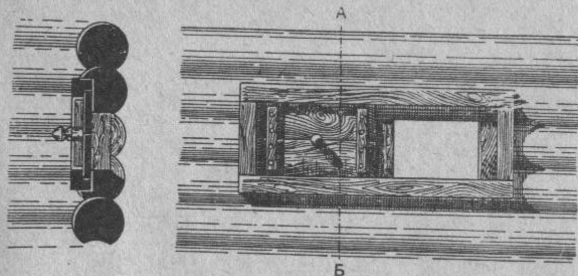
Схема устройства волокового окна
