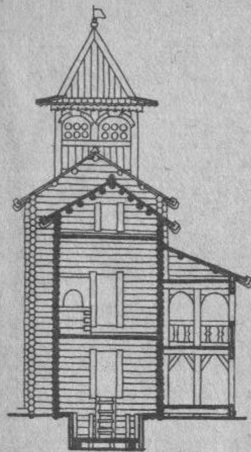
Реконструкция того же терема. Слева — поперечный разрез с восточной стороны, справа — вид с севера. Важным мотивом композиции терема была галерея. Арочные галереи неизменно повторяются в произведениях прикладного искусства, книжной миниатюре, палатном письме икон и фресок
