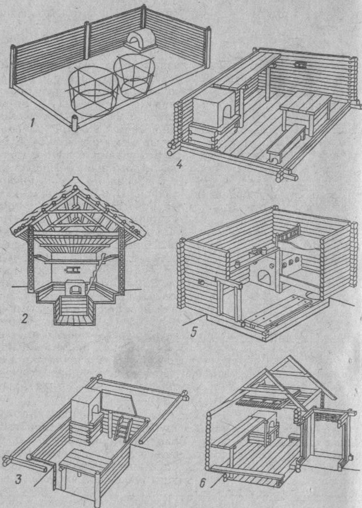
Типы наземных изб без подполий. 1 — двухкамерная постройка с хозяйственными ямами; 2 — изба с земляными лавками по периметру стен, стратиграфические наблюдения позволяют реконструировать потолки («подволока», «подволока»), которые старались утеплить; 3 — жилище с заглубленной центральной частью; 4—5 — избы с полами.
