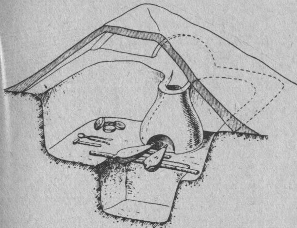
Реконструкция домницы для выплавки железа. Над предгорновой ямой лежат воздуходувные мехи. Здесь же инструменты металлурга — молоток, клещи. Крицы имеют круглую форму. Рисунок из книги: Колчин Б. А. Черная металлургия и металлообработка в Древней Руси. М., 1953
