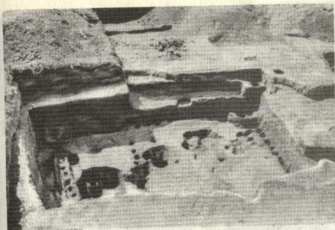
Мастерская по выплавке железа. Плетневые стены, от которых сохранились следы столбиков, были обмазаны глиной. Мастерская разделена на два помещения. В одном из них находился сильно разрушенный горн, перед ним хорошо видна яма. В заполнении найдено много железного шлака.
