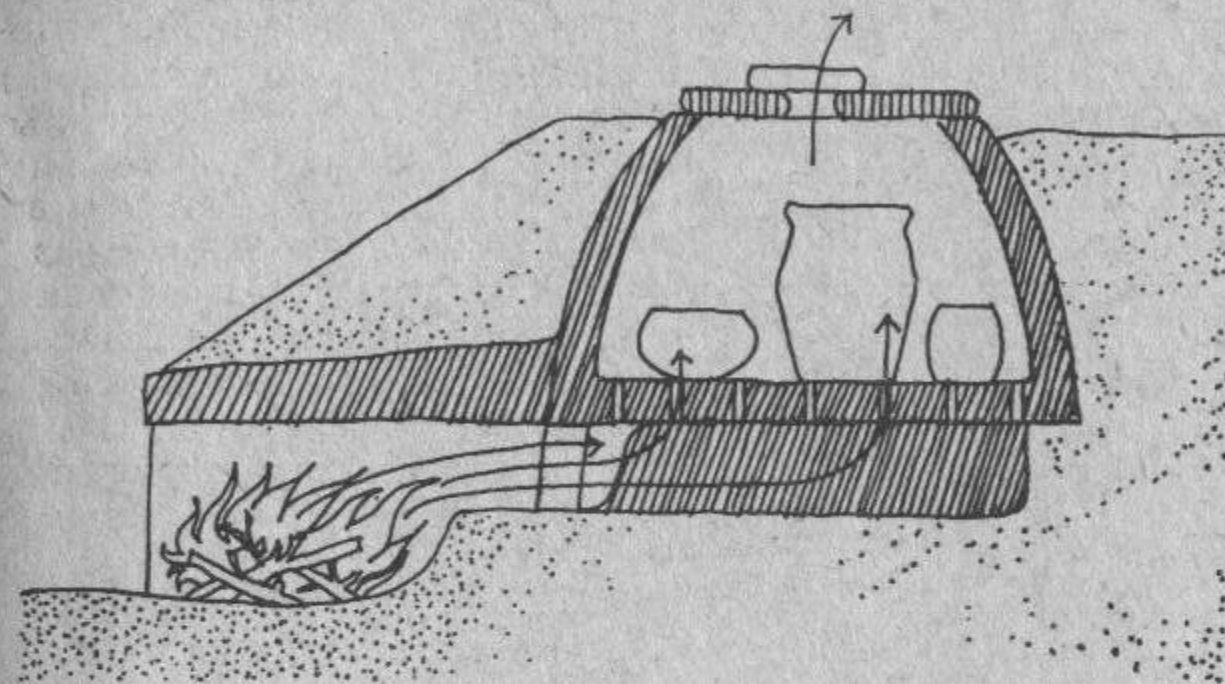
Реконструкция гончарного горна для обжига посуды
