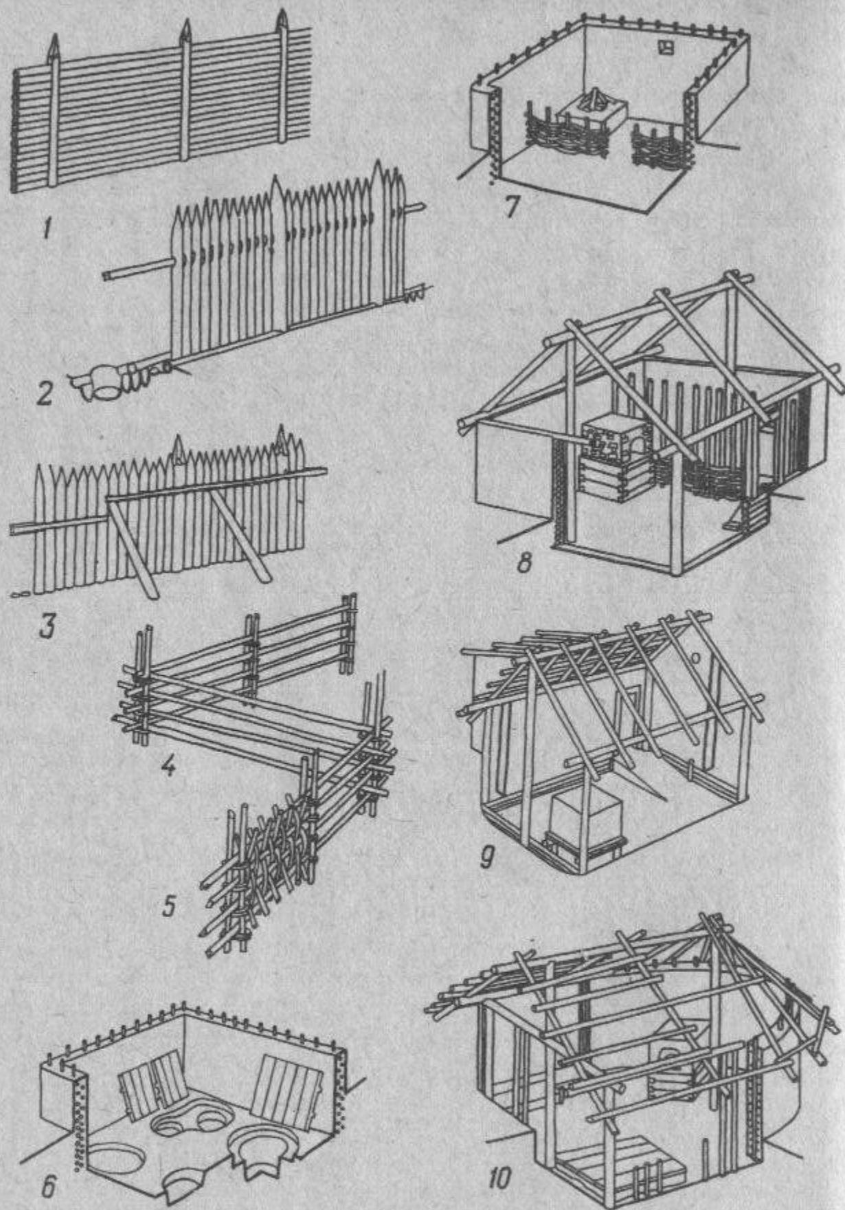
Типы оград и постройки каркасной конструкции по материалам раскопок в Рязани. 1 — забор-оплот: бревна-заплогины забирались в пазы вертикальных столбов; 2 — частокол; 3 — частокол с подпорками-раскосами; 4 — ограда из парных столбиков с горизонтальными
