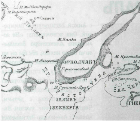
Остров Колчак на карте южной части Таймырского залива
